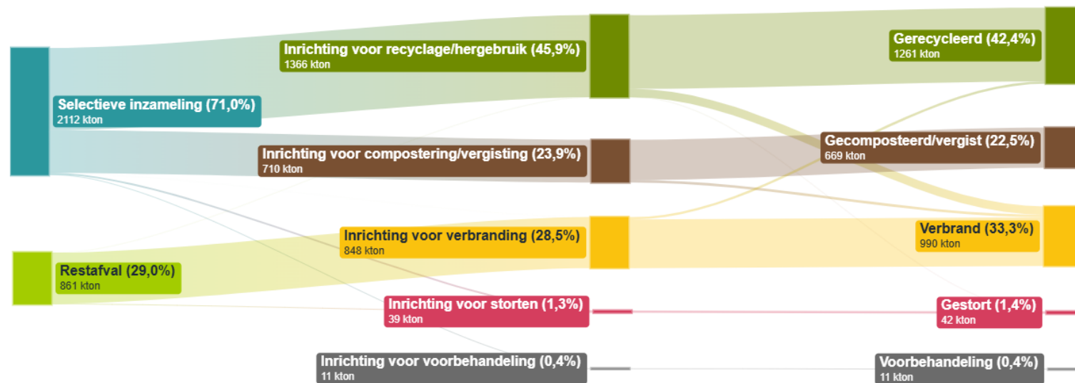
Figuur 3: Stroomdiagram met aanduiding van de inrichting voor verwerking van het huishoudelijk afval in Vlaanderen en de effectieve verwerking in 2024 (hoeveelheden in kton).
