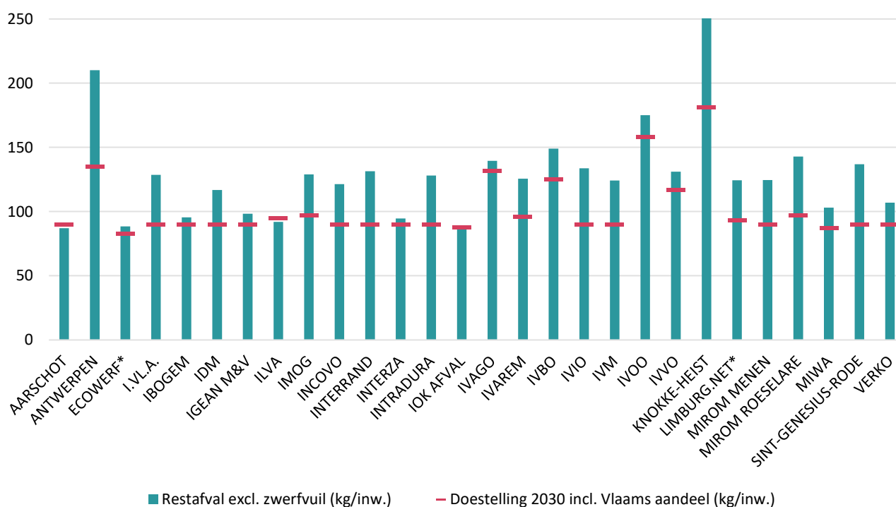
Figuur 10. Het restafvalcijfer (exclusief zwerfvuil) per intercommunale in 2024 ten opzichte van hun doelstelling in 2030 (inclusief het Vlaams aandeel).
