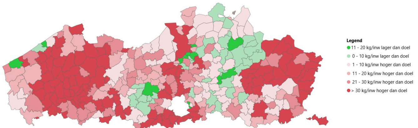
Figuur 11. Afstand van het restafvalcijfer per gemeente (exclusief zwerfvuil) in 2024 ten opzichte van hun doelstelling in 2030 (inclusief het Vlaams aandeel).
