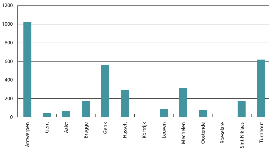
Oppervlakte met effectief natuurbeheer, in 2010, in ha.
