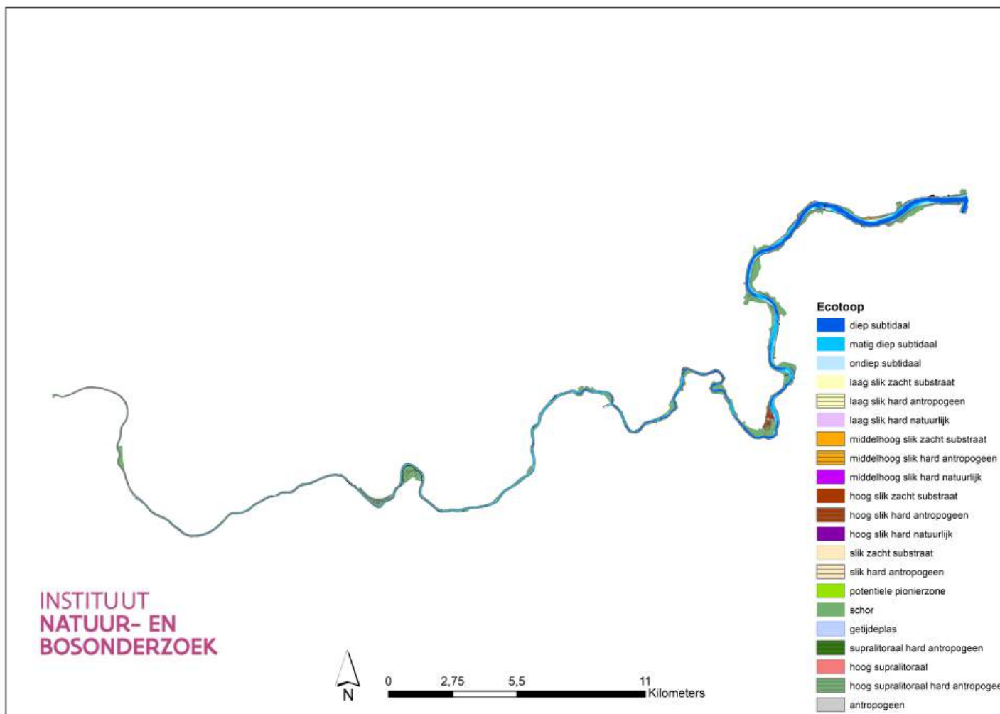
Figuur 3.6: Ecotopenkaart 2022 Boven-Zeeschelde 1.0
