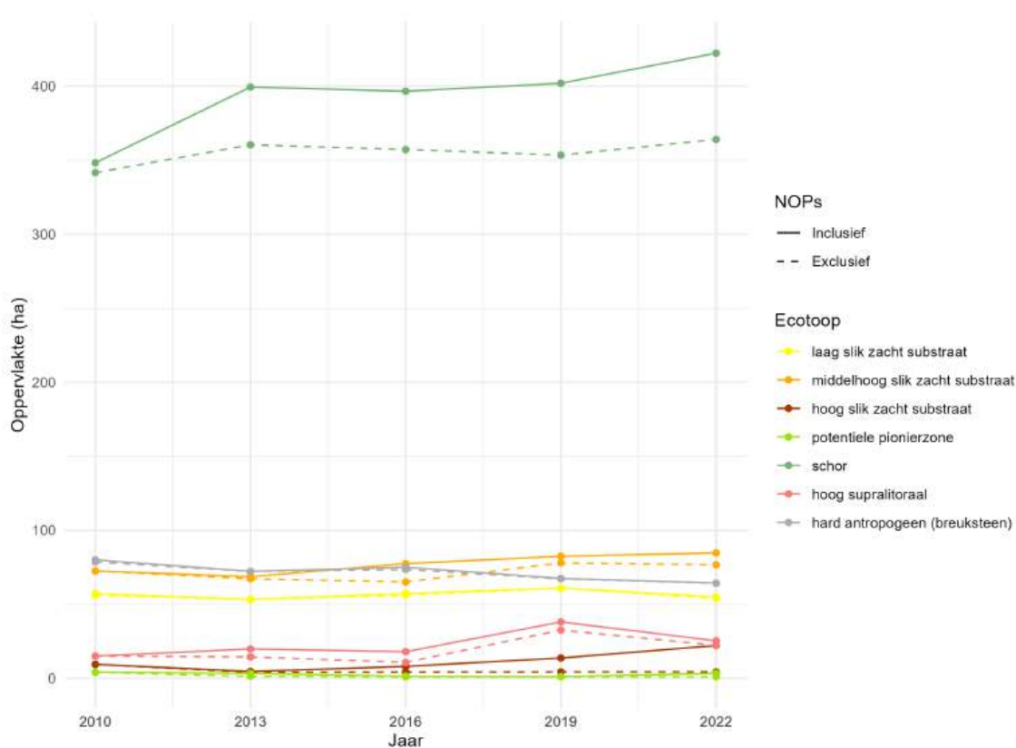
Figuur 3.7: Temporele evolutie van de oppervlakte van de ecologisch belangrijke ecotopen Zeeschelde 1.0 in de Boven-Zeeschelde met en zonder NOP's (natuurontwikkelingsprojecten zoals ontpolderingen, GGG's en dijkverleggingen)
