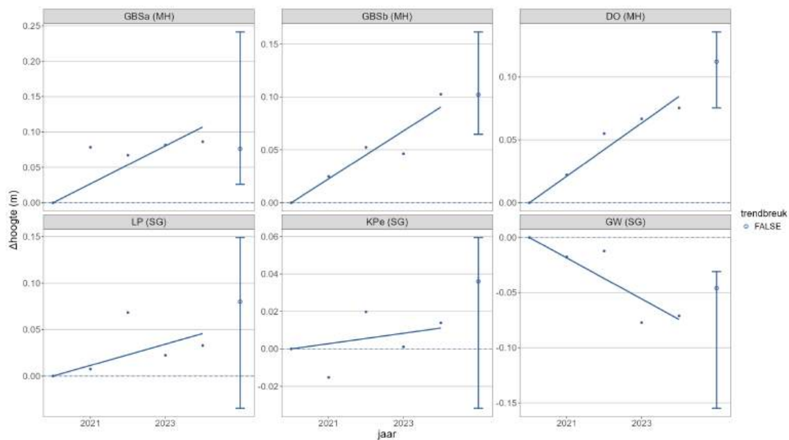
Figuur 12.3: Trends (2020 - 2024) en trendbreuken (2025; 95% betrouwbaarheidsinterval) op de scorplaatens in de Beneden Zeeschelde.
