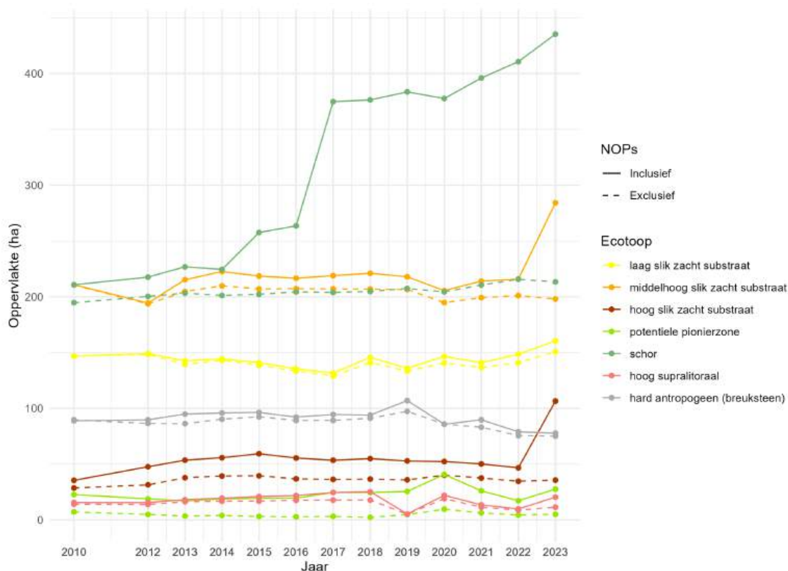
Figuur 3.4: Temporele evolutie van de oppervlakte van de ecologisch belangrijke ecotopen Zeeschelde 1.0 in de Beneden-Zeeschelde met en zonder NOP's (natuurontwikkelingsprojecten zoals ontponderingen, GGG's en dijkverleggingen)
