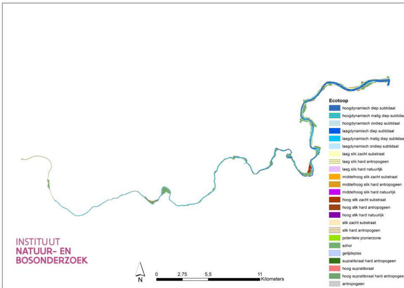
Figuur 3.8: Ecotopenkaart 2022 Boven-Zeeschelde 2.0
