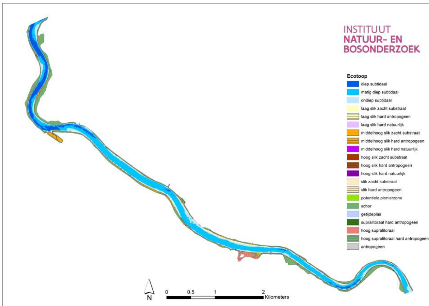
Figuur 3.9: Ecotopenkaart 2022 Rupel 1.0
