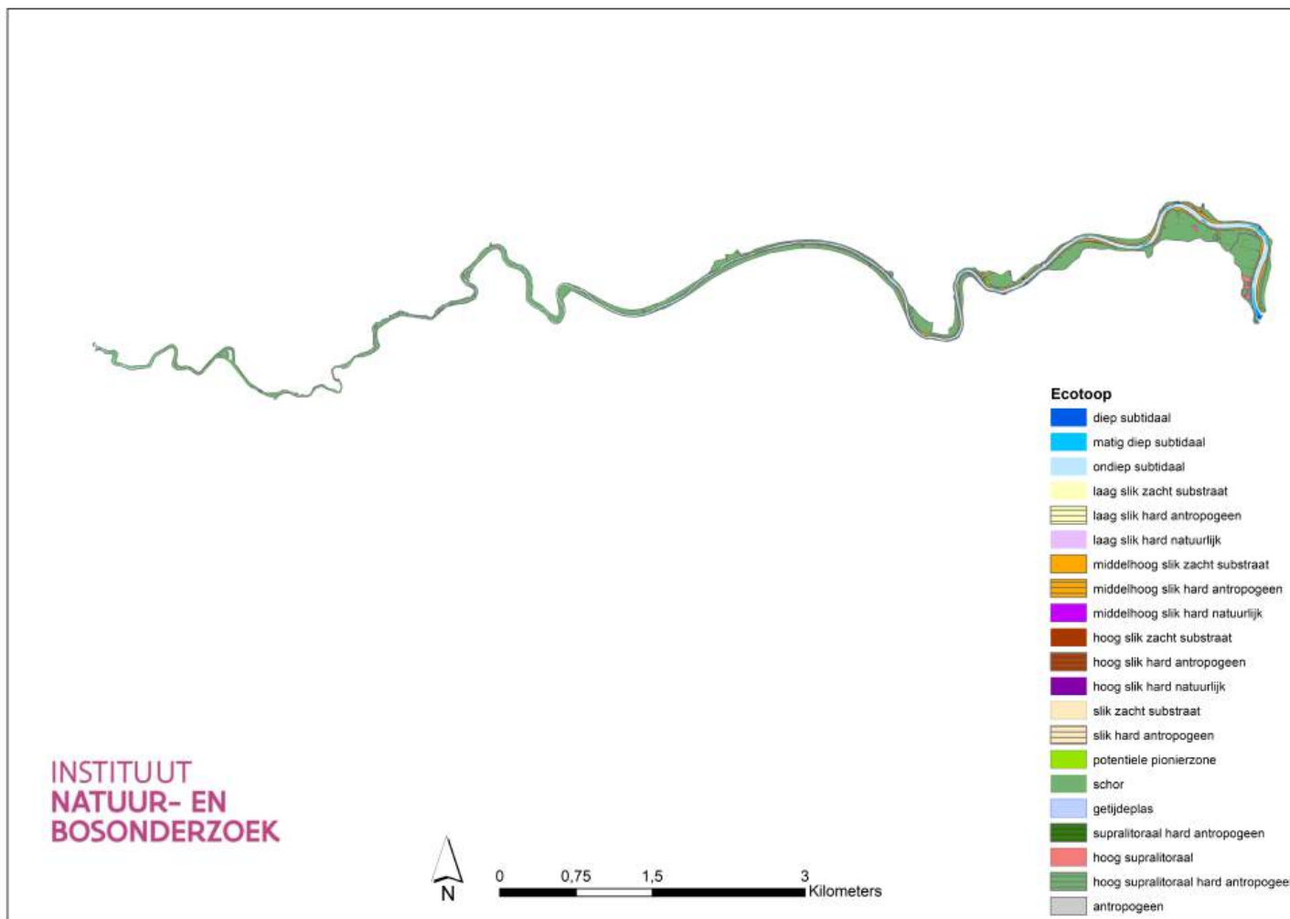
Figuur 3.11: Ecotopenkaart 2022 Durme 1.0
