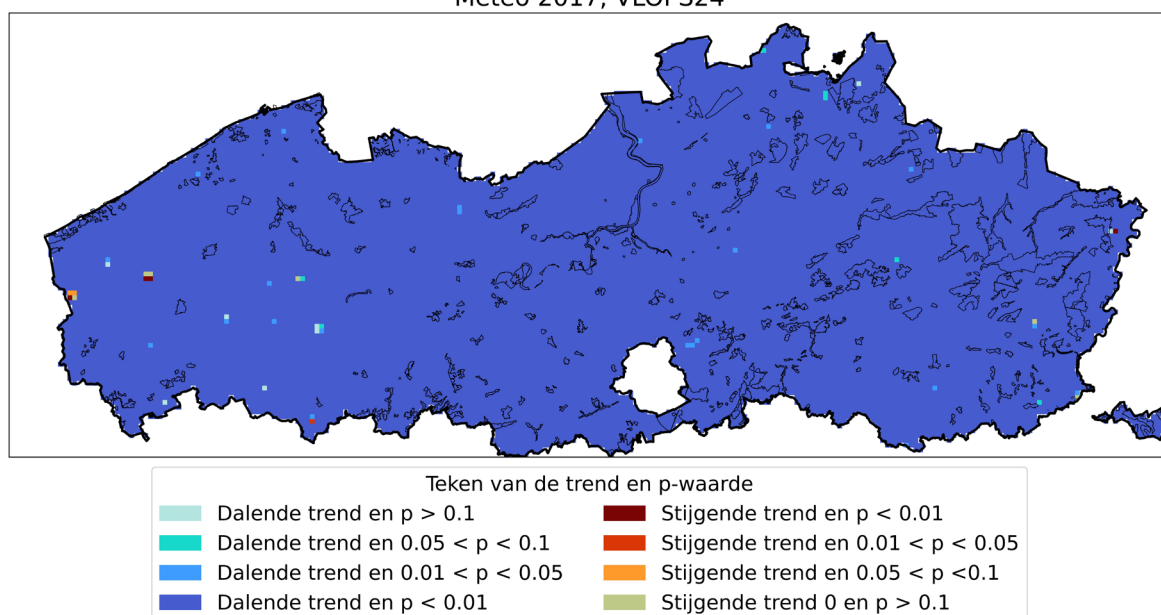
Totale Vlaamse NO y -deposities Meteo 2017, VLOPS24
