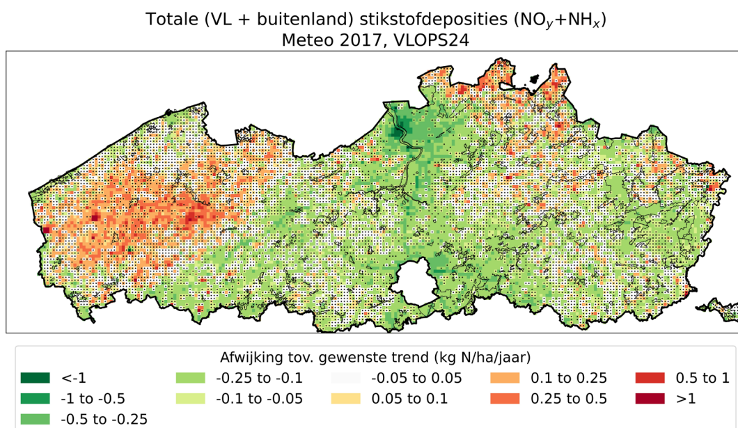
Figuur 47: Afwijking tussen de geobserveerde jaarlijkse lineaire trend in de periode 2015 – 2022 en de gewenste jaarlijkse lineaire trend op basis van de evolutie tussen 2015 en het toetspunt 2030 voor de totale (VL + buitenland) jaarlijkse stikstofdeposities ( \text{NO}_y + \text{NH}_x ) op 1 km bij 1 km resolutie in de periode, zoals gemodelleerd door het VLOPS model. Positieve waarden (rode locaties) duiden op locaties waar de gewenste trend een grotere daling / kleinere stijging voorziet dan de geobserveerde trend, en dus op locaties waar de doelstelling 2030 bij een aangehouden lineaire trend niet gehaald wordt. Negatieve waarden / groene locaties duiden het omgekeerde gedrag aan. Gridcellen met zwarte punten in duiden op locaties waar de afwijking tussen beide trends niet significant is ( p > 0.05 ). De dikke zwarte lijn geeft de buitengrenzen van Vlaanderen weer, de dunne lijnen de locaties van de Habitatrichtlijngebieden (SBZ-H).
