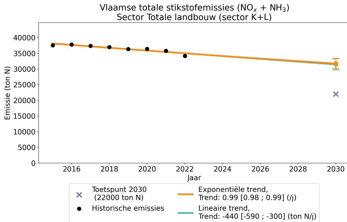
Figuur 14: Verloop van de jaarlijkse totale stikstofemissies ( \text{NO}_x + \text{NH}_3 ) voor de sector Totale landbouw (sector K+L) in Vlaanderen (in ton N). Zwarte punten: gerapporteerde jaarlijkse emissies voor de historische jaren. Groene en oranje lijn: lineaire respectievelijk exponentiële regressie door de punten voor de periode 2015-2022. Groene en oranje punt in 2030: projectie van de emissies volgens een lineaire respectievelijke exponentiële trend, met betrouwbaarheidsinterval (2-sigma onzekerheid). Paarse kruis: toetspunt voor 2030.
