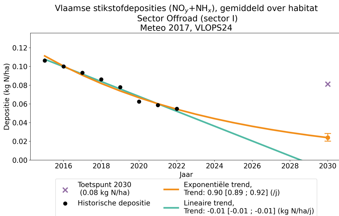
Figuur 41: Verloop van de jaarlijkse Vlaamse stikstofdeposities ( \text{NO}_y + \text{NH}_x ) gemiddeld over habitats in Vlaanderen voor de sector Offroad (sector I) (in kg N/ha/j). Zwarte punten: gemodelleerde jaarlijkse deposities voor de historische jaren. Groene en oranje lijn: lineaire respectievelijk exponentiële regressie door de punten. Groene en oranje punt in 2030: projectie van de depositie volgens een lineaire respectievelijk exponentiële trend, met betrouwbaarheidsinterval (2-sigma onzekerheid). Paarse kruis: toetspunt voor 2030.
