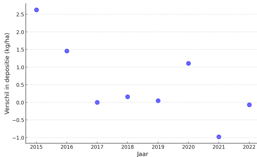
Figuur 58: Impact van het gebruik van jaarspecifieke meteo in plaats van meteo 2017. De plot toont het verschil in de jaarlijkse totale (Vlaanderen + buitenland) N-depositie ( \text{NO}_x + \text{NH}_x ) gemiddeld over de Vlaamse habitats op basis van VLOPS24, tussen enerzijds een berekening op basis van meteo 2017 en anderzijds de jaarspecifieke meteo. Positieve waarden: de depositie berekend op basis van de jaarspecifieke meteo is lager dan deze bij meteo 2017. De plot toont, net zoals alle andere plots in dit rapport, de resultaten na kalibratie.
