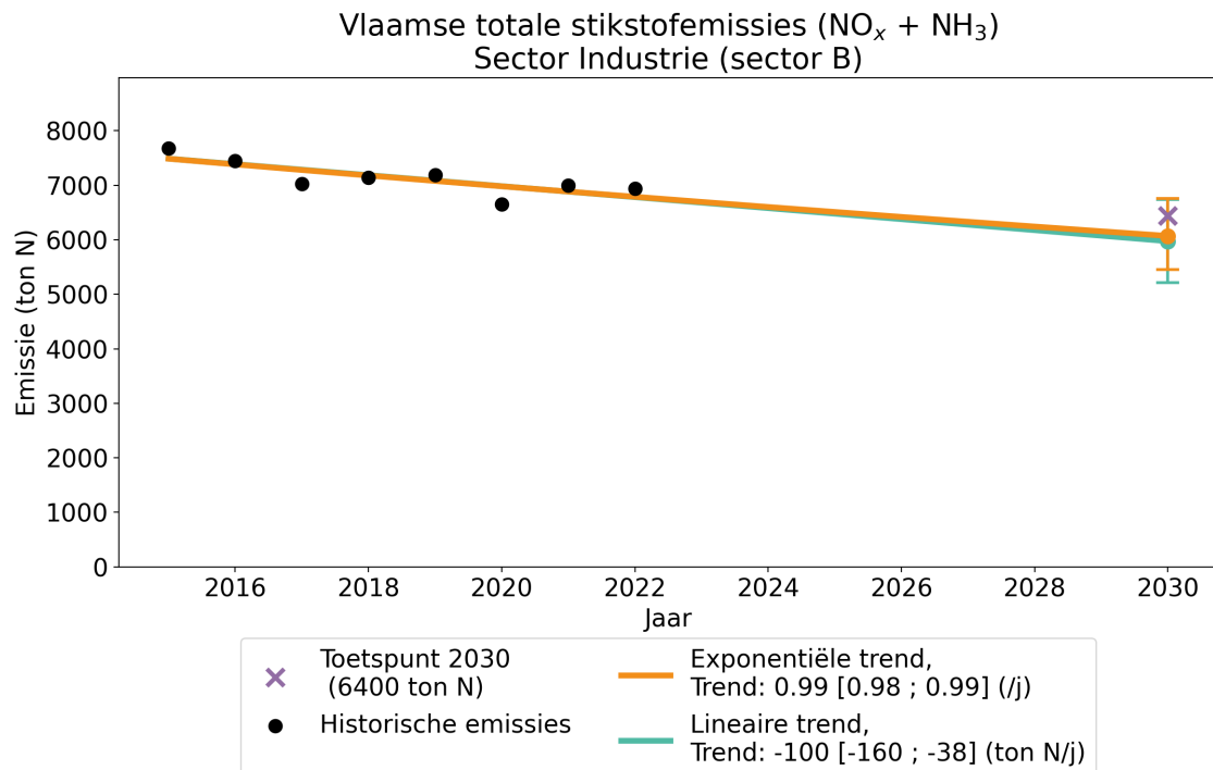
Figuur 5: Verloop van de jaarlijkse totale stikstofemissies ( \text{NO}_x + \text{NH}_3 ) voor de sector Industrie (sector B) in Vlaanderen (in ton N). Zwarte punten: gerapporteerde jaarlijkse emissies voor de historische jaren. Groene en oranje lijn: lineaire respectievelijk exponentiële regressie door de punten voor de periode 2015-2022. Groene en oranje punt in 2030: projectie van de emissies volgens een lineaire respectievelijke exponentiële trend, met betrouwbaarheidsinterval (2-sigma onzekerheid). Paarse kruis: toetspunt voor 2030.
