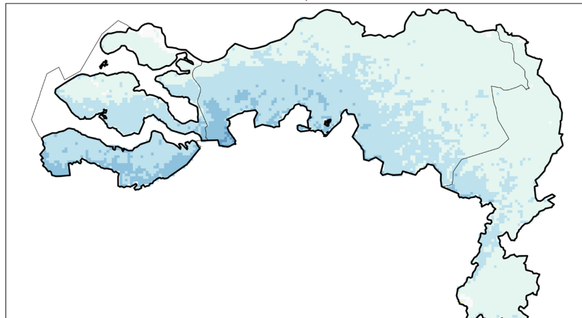
Totale Vlaamse stikstofdeposities ( \text{NO}_y + \text{NH}_x ) op Zuid-Nederland Meteo 2017, VLOPS24
