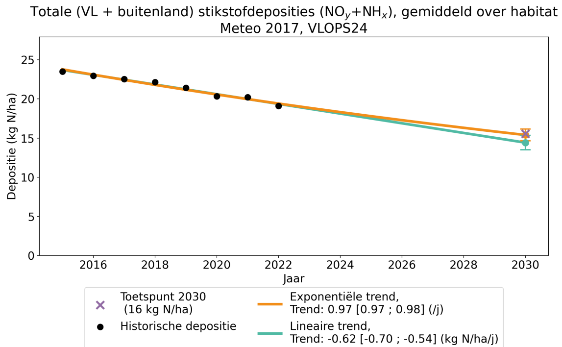
Figuur 28: Verloop van de totale (VL + buitenland) jaarlijkse stikstofdeposities ( \text{NO}_y + \text{NH}_x ) gemiddeld over habitats in Vlaanderen (in kgN/ha/j). Zwarte punten: gerapporteerde jaarlijkse deposities voor de historische jaren. Groene en oranje lijn: lineaire respectievelijk exponentiële regressie door de punten. Groene en oranje punt in 2030: projectie van de deposities volgens een lineaire respectievelijke exponentiële trend, met betrouwbaarheidsinterval (2-sigma onzekerheid). Paarse kruis: toetspunt voor 2030.
