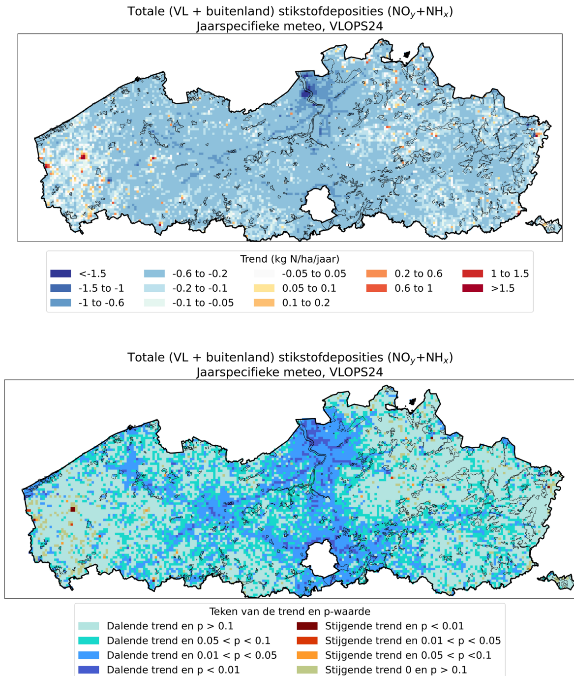
Figuur 60: Lineaire trend van de totale (VL + buitenland) jaarlijkse stikstofdeposities ( \text{NO}_y + \text{NH}_x ) op 1 km bij 1 km resolutie in de periode 2015 – 2022, zoals gemodelleerd door het VLOPS model, indien voor elk jaar gebruik gemaakt wordt van de meteo voor dat jaar. De bovenste figuur geeft de jaarlijkse trend (in kg/ha/jaar), de onderste figuur visualiseert het teken van de trend en de p-waarde in één figuur. Deze figuur is de tegenhanger van Figuur 46, maar dan op basis van jaarspecifieke meteorologie.
