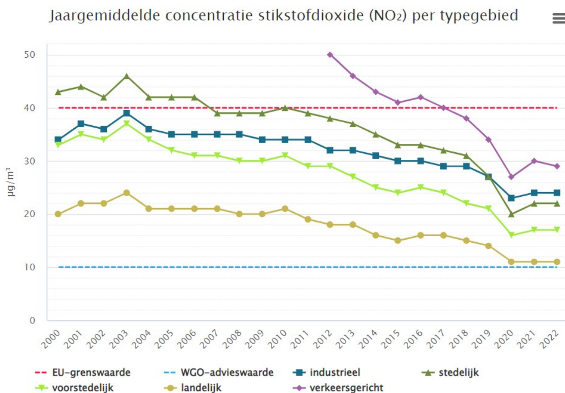
Figuur 61: Evolutie van de jaargemiddelde NO 2 -concentratie per typegebied (in µg/m 3 ). Bron: https://www.vmm.be/lucht/stikstof/concentratie-stikstofdioxide .
