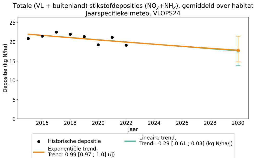
Figuur 59: Verloop van de totale (VL + buitenland) jaarlijkse stikstofdeposities ( \text{NO}_y + \text{NH}_x ) gemiddeld over habitats in Vlaanderen (in kg N/ha/j), indien voor elk jaar gebruik gemaakt wordt van de meteo voor dat jaar. Zwarte punten: gerapporteerde jaarlijkse deposities voor de historische jaren. Groene en oranje lijn: lineaire respectievelijk exponentiële regressie door de punten. Groene en oranje punt in 2030: projectie van de deposities volgens een lineaire respectievelijke exponentiële trend, met betrouwbaarheidsinterval (2-sigma onzekerheid). Paarse kruis: toetspunt voor 2030. Deze figuur is de tegenhanger van Figuur 28, maar dan op basis van jaarspecifieke meteorologie.
