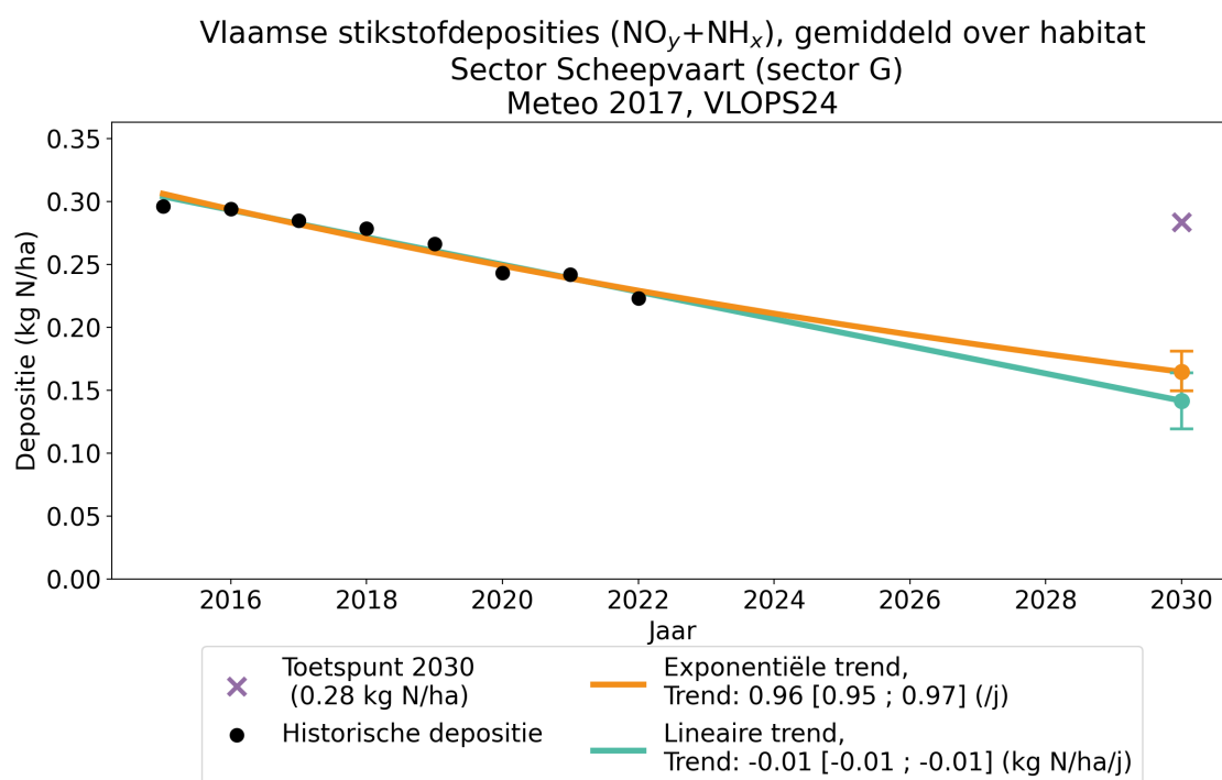
Figuur 39: Verloop van de jaarlijkse Vlaamse stikstofdeposities ( \text{NO}_y + \text{NH}_x ) gemiddeld over habitats in Vlaanderen voor de sector Scheepvaart (sector G) (in kg N/ha/j). Zwarte punten: gemodelleerde jaarlijkse deposities voor de historische jaren. Groene en oranje lijn: lineaire respectievelijk exponentiële regressie door de punten. Groene en oranje punt in 2030: projectie van de depositie volgens een lineaire respectievelijke exponentiële trend, met betrouwbaarheidsinterval (2-sigma onzekerheid). Paarse kruis: toetspunt voor 2030.
