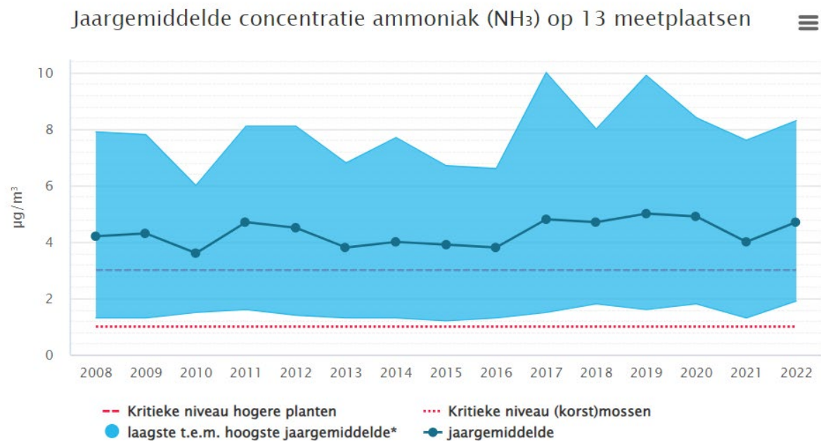
Figuur 62: Evolutie van de jaargemiddelde NH 3 -concentratie op basis van de metingen (in \mu\text{g}/\text{m}^3 ). De blauwe zone bakent het gebied af waarbinnen de jaargemiddelde concentraties van de individuele meetplaatsen zich bevinden.
