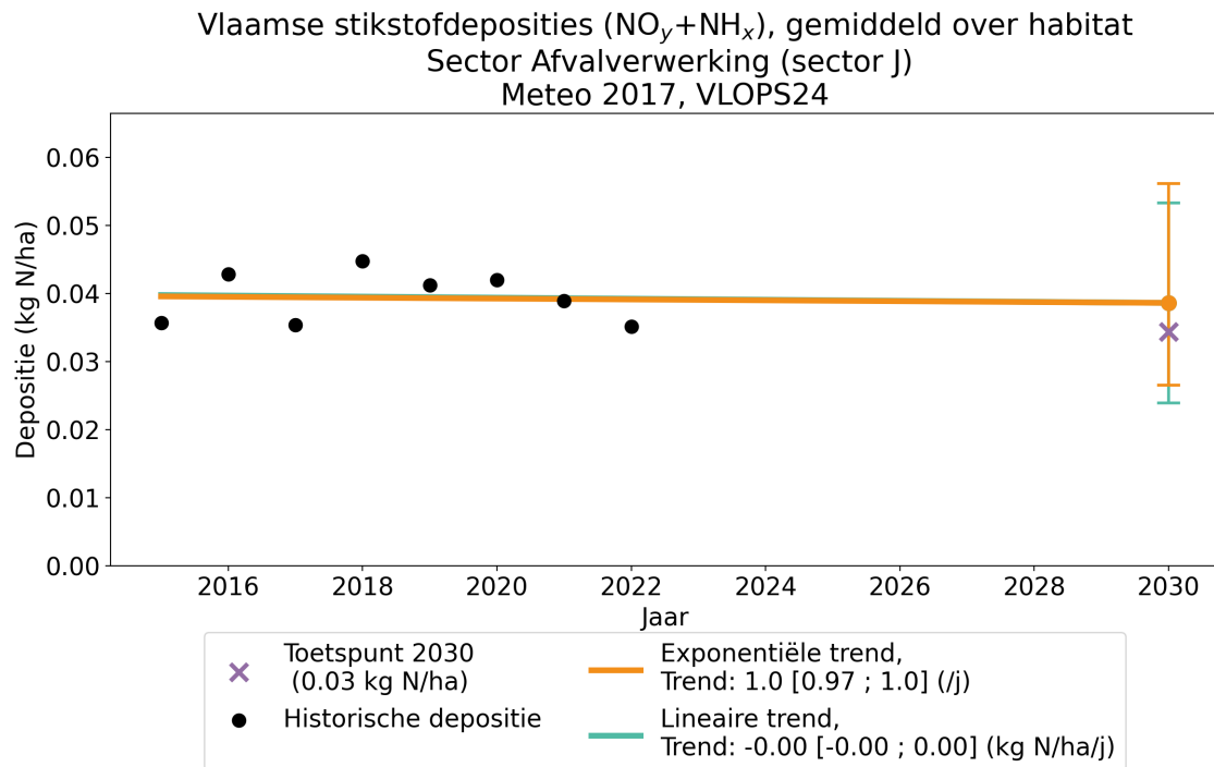
Figuur 45: Verloop van de jaarlijkse Vlaamse stikstofdeposities ( \text{NO}_y + \text{NH}_x ) gemiddeld over habitats in Vlaanderen voor de sector Afvalverwerking (sector J) (in kg N/ha/j). Zwarte punten: gemodelleerde jaarlijkse deposities voor de historische jaren. Groene en oranje lijn: lineaire respectievelijk exponentiële regressie door de punten. Groene en oranje punt in 2030: projectie van de depositie volgens een lineaire respectievelijke exponentiële trend, met betrouwbaarheidsinterval (2-sigma onzekerheid). Paarse kruis: toetspunt voor 2030.
