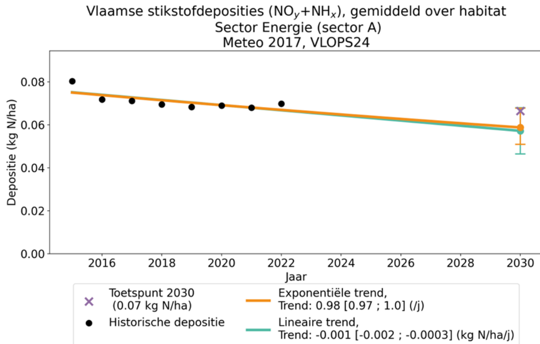
Figuur 35: Verloop van de jaarlijkse Vlaamse stikstofdeposities ( \text{NO}_y + \text{NH}_x ) gemiddeld over habitats in Vlaanderen voor de sector Energie (sector A) (in kg N/ha/j). Zwarte punten: gemodelleerde jaarlijkse deposities voor de historische jaren. Groene en oranje lijn: lineaire respectievelijk exponentiële regressie door de punten. Groene en oranje punt in 2030: projectie van de depositie volgens een lineaire respectievelijke exponentiële trend, met betrouwbaarheidsinterval (2-sigma onzekerheid). Paarse kruis: toetspunt voor 2030.
