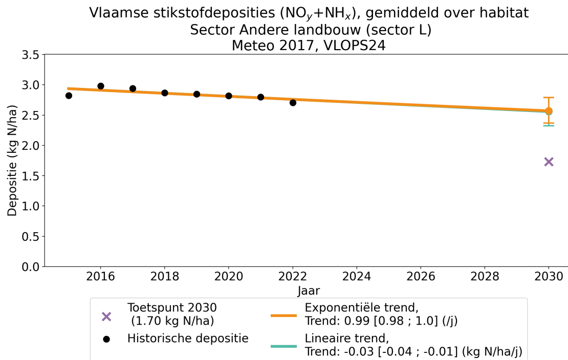
Figuur 43: Verloop van de jaarlijkse Vlaamse stikstofdeposities ( \text{NO}_y + \text{NH}_x ) gemiddeld over habitats in Vlaanderen voor de sector Andere landbouw (sector L) (in kg N/ha/j). Zwarte punten: gemodelleerde jaarlijkse deposities voor de historische jaren. Groene en oranje lijn: lineaire respectievelijk exponentiële regressie door de punten. Groene en oranje punt in 2030: projectie van de depositie volgens een lineaire respectievelijke exponentiële trend, met betrouwbaarheidsinterval (2-sigma onzekerheid). Paarse kruis: toetspunt voor 2030.
