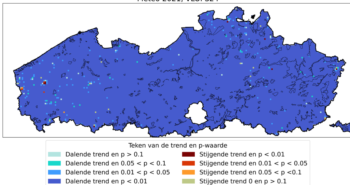
Totale (VL + buitenland) stikstofdeposities ( \text{NO}_y + \text{NH}_x ) Meteo 2021, VLOPS24
