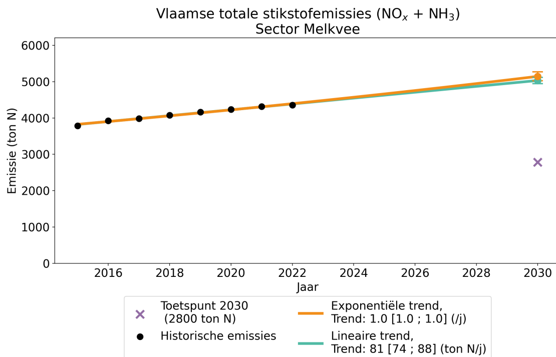
Figuur 17: Verloop van de jaarlijkse totale stikstofemissies ( \text{NO}_x + \text{NH}_3 ) voor de sector Melkvee in Vlaanderen (in ton N). Zwarte punten: gerapporteerde jaarlijkse emissies voor de historische jaren.
