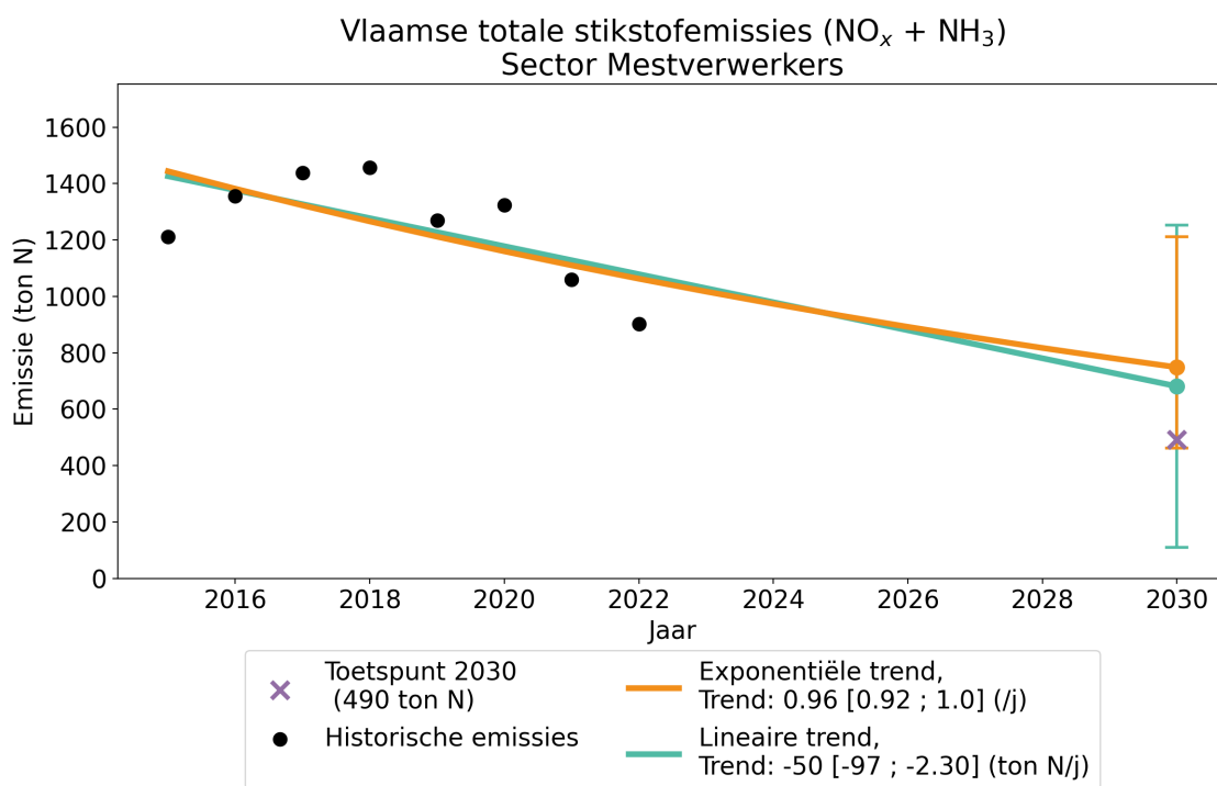
Figuur 25: Verloop van de jaarlijkse totale stikstofemissies ( \text{NO}_x + \text{NH}_3 ) voor de sector Mestverwerkers in Vlaanderen (in ton N). Zwarte punten: gerapporteerde jaarlijkse emissies voor de historische jaren. Groene en oranje lijn: lineaire respectievelijk exponentiële regressie door de punten voor de periode 2015-2022. Groene en oranje punt in 2030: projectie van de emissies volgens een lineaire respectievelijke exponentiële trend, met betrouwbaarheidsinterval (2-sigma onzekerheid). Paarse kruis: toetspunt voor 2030.
