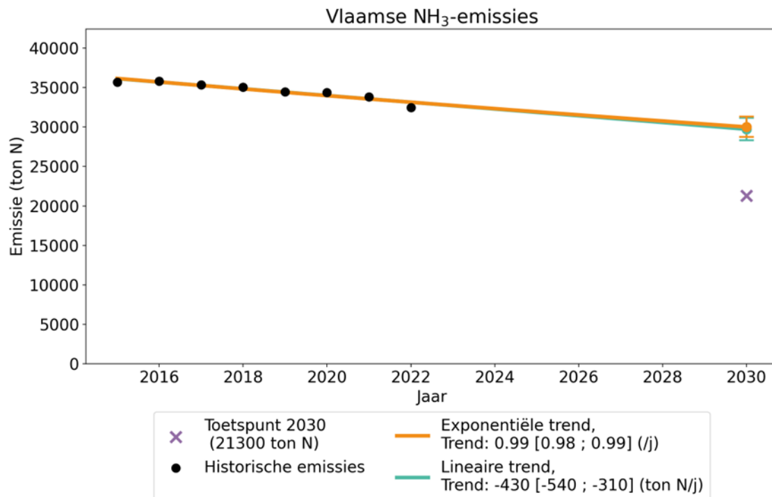
Figuur 3: Verloop van de totale jaarlijkse Vlaamse NH 3 -emissies (in ton N). Zwarte punten: gerapporteerde jaarlijkse emissies voor de historische jaren. Groene en oranje lijn: lineaire respectievelijk exponentiële regressie door de punten voor de periode 2015-2022. Groene en oranje punt in 2030: projectie van de emissies volgens een lineaire respectievelijk exponentiële trend, met betrouwbaarheidsinterval (2-sigma onzekerheid). Paarse kruis: toetspunt voor 2030.
