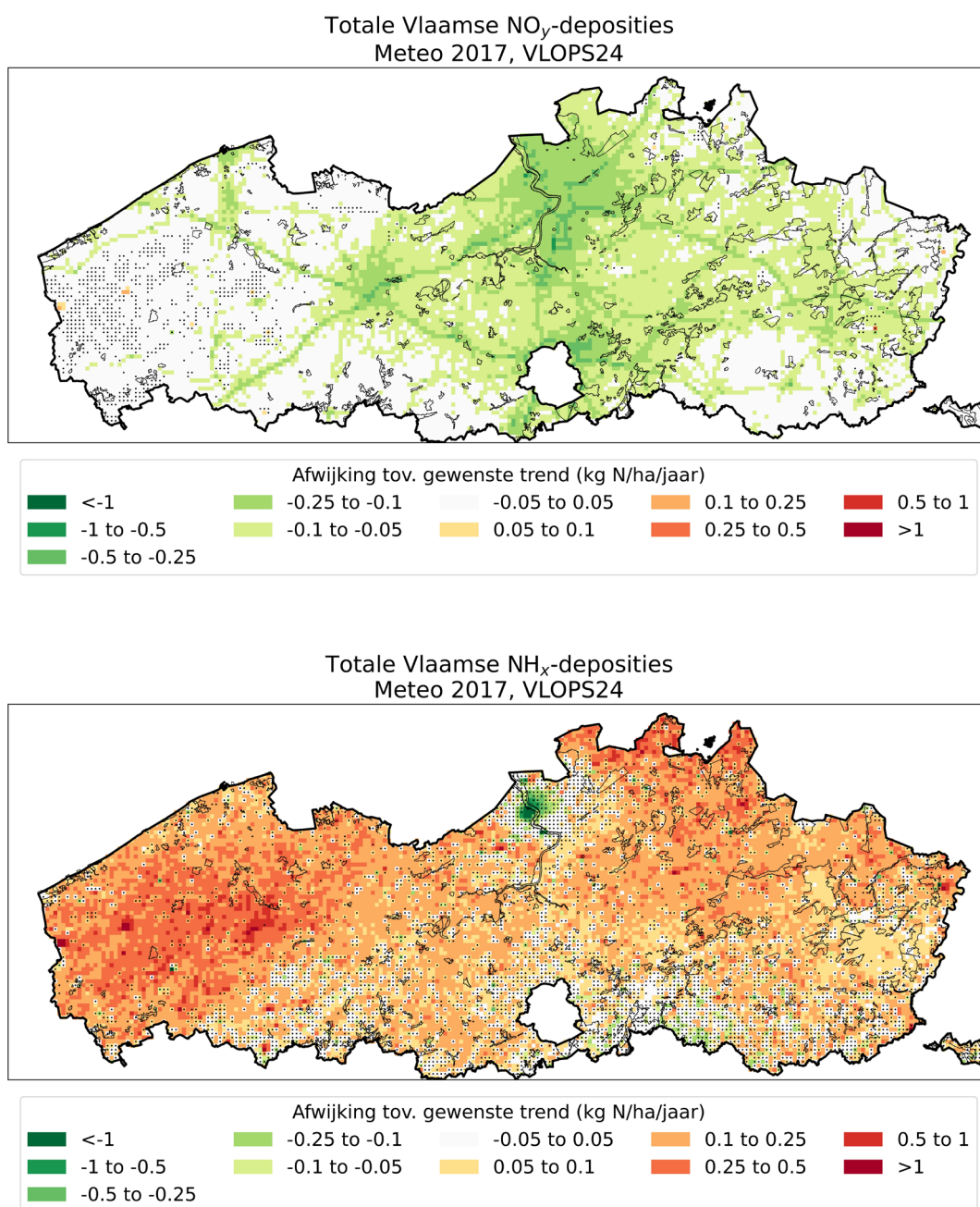
Figuur 52: Afwijking tussen de geobserveerde jaarlijkse lineaire trend in de periode 2015 – 2022 en de gewenste jaarlijkse lineaire trend op basis van de evolutie tussen 2015 en het toetspunt 2030 voor de Vlaamse jaarlijkse NO y (bovenste figuur) en NH x (onderste figuur) depositie op 1 km bij 1 km resolutie in de periode, zoals gemodelleerd door het VLOPS model. Positieve waarden (rode locaties) duiden op locaties waar de gewenste trend een grotere daling / kleinere stijging voorziet dan de geobserveerde trend, en dus op locaties waar de doelstelling 2030 bij een aangehouden lineaire trend niet gehaald wordt. Negatieve waarden / groene locaties duiden het omgekeerde gedrag aan. Gridcellen met zwarte punten in duiden op locaties waar de afwijking tussen beide trends niet significant is ( p > 0.05 ). De dikke zwarte lijn geeft de buitengrenzen van Vlaanderen weer, de dunne lijnen de locaties van de Natura 2000 gebieden.
