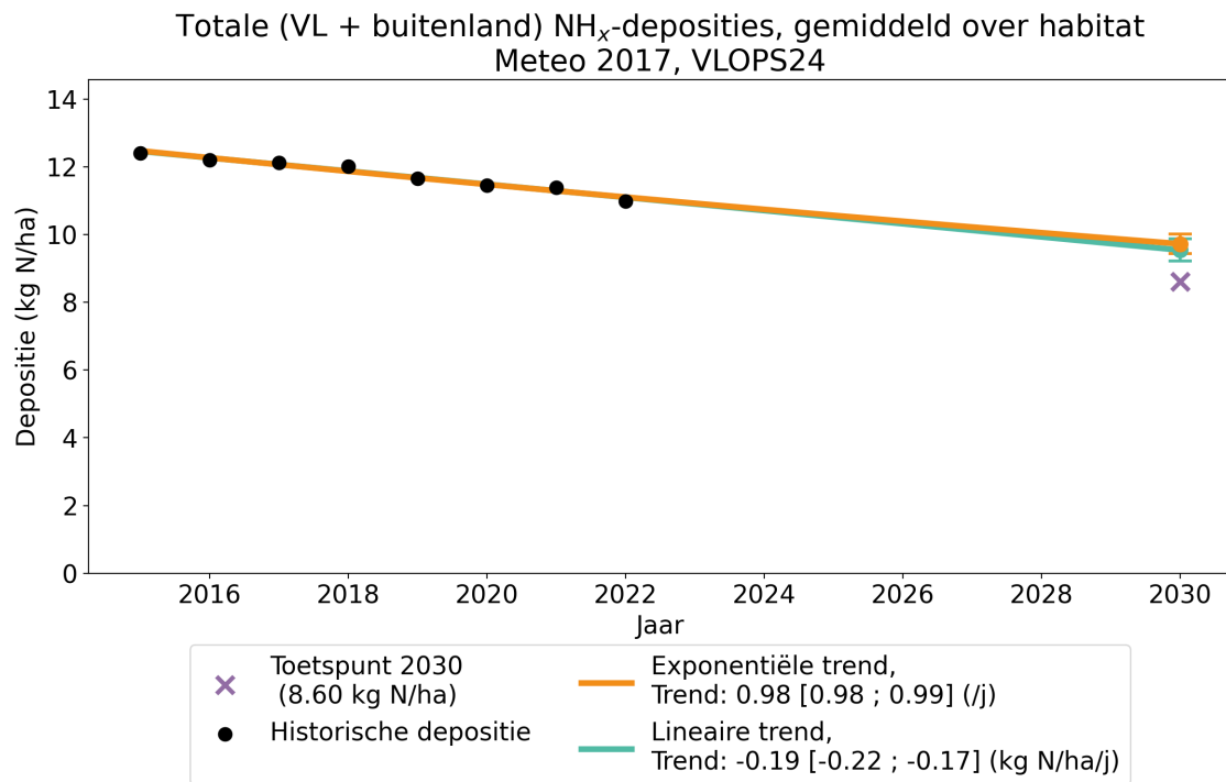
Figuur 30: Verloop van de totale (VL + buitenland) jaarlijkse \text{NH}_x -deposities gemiddeld over habitats in Vlaanderen (in kg N/ha/j). Zwarte punten: gerapporteerde jaarlijkse deposities voor de historische jaren. Groene en oranje lijn: lineaire respectievelijk exponentiële regressie door de punten. Groene en oranje punt in 2030: projectie van de deposities volgens een lineaire respectievelijk exponentiële trend, met betrouwbaarheidsinterval (2-sigma onzekerheid). Paarse kruis: toetspunt voor 2030.
