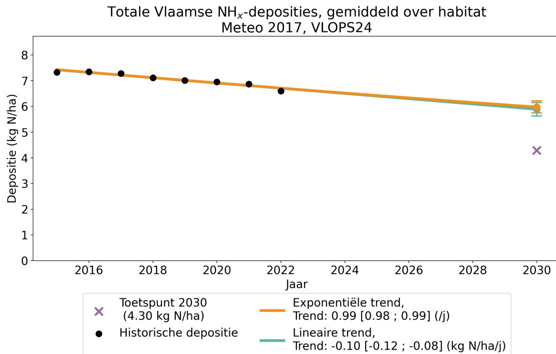
Figuur 33: Verloop van de jaarlijkse Vlaamse \text{NH}_x -deposities gemiddeld over habitats in Vlaanderen (in kg N/ha/j). Zwarte punten: gerapporteerde jaarlijkse deposities voor de historische jaren. Groene en oranje lijn: lineaire respectievelijk exponentiële regressie door de punten. Groene en oranje punt in 2030: projectie van de deposities volgens een lineaire respectievelijke exponentiële trend, met betrouwbaarheidsinterval (2-sigma onzekerheid). Paarse kruis: toetspunt voor 2030.
