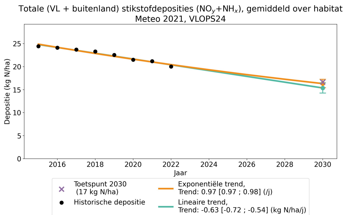
Figuur 56: Verloop van de totale (VL + buitenland) jaarlijkse stikstofdeposities ( \text{NO}_y + \text{NH}_x ) gemiddeld over habitats in Vlaanderen (in kg N/ha), indien voor elk jaar gebruik gemaakt wordt van de meteo van 2021. Zwarte punten: gerapporteerde jaarlijkse deposities voor de historische jaren. Groene en oranje lijn: lineaire respectievelijk exponentiële regressie door de punten. Groene en oranje punt in 2030: projectie van de deposities volgens een lineaire respectievelijk exponentiële trend, met betrouwbaarheidsinterval (2-sigma onzekerheid). Paarse kruis: toetspunt voor 2030. Deze figuur is de tegenhanger van Figuur 28, maar dan op basis van meteo 2021.
