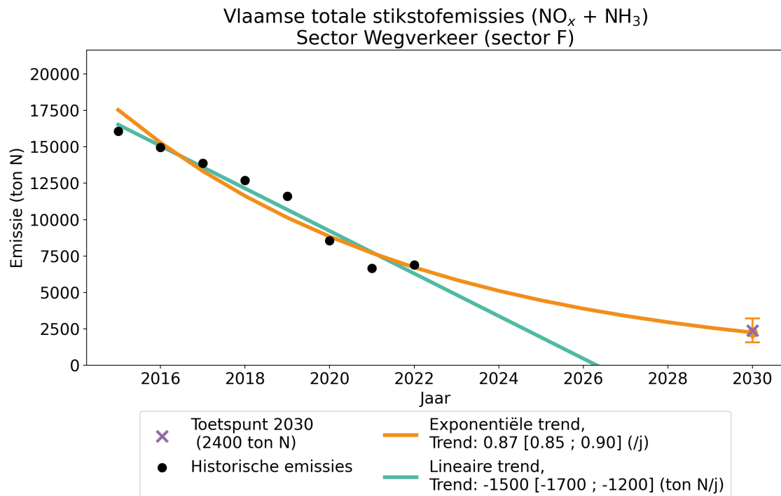
Figuur 8: Verloop van de jaarlijkse totale stikstofemissies ( \text{NO}_x + \text{NH}_3 ) voor de sector Wegverkeer (sector F) in Vlaanderen (in ton N). Zwarte punten: gerapporteerde jaarlijkse emissies voor de historische jaren. Groene en oranje lijn: lineaire respectievelijk exponentiële regressie door de punten voor de periode 2015-2022. Groene en oranje punt in 2030: projectie van de emissies volgens een lineaire respectievelijk exponentiële trend, met betrouwbaarheidsinterval (2-sigma onzekerheid). Paarse kruis: toetspunt voor 2030.
