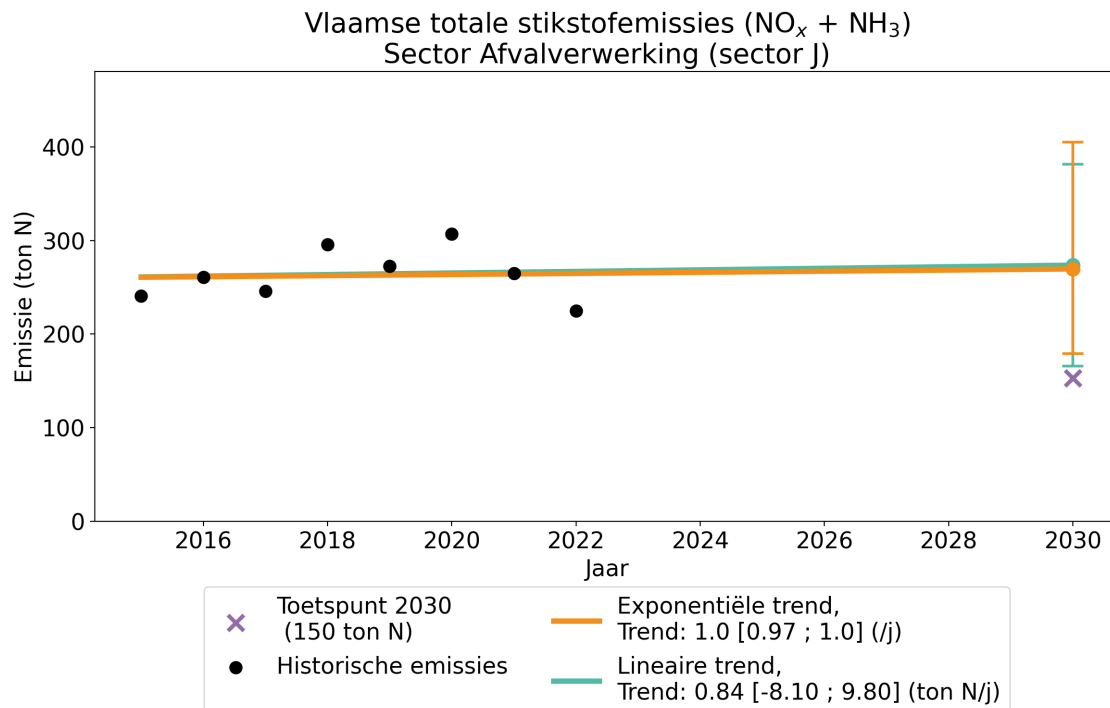
Figuur 16: Verloop van de jaarlijkse totale stikstofemissies ( \text{NO}_x + \text{NH}_3 ) voor de sector Afvalverwerking (sector J) in Vlaanderen (in ton N). Zwarte punten: gerapporteerde jaarlijkse emissies voor de historische jaren. Groene en oranje lijn: lineaire respectievelijk exponentiële regressie door de punten voor de periode 2015-2022. Groene en oranje punt in 2030: projectie van de emissies volgens een lineaire respectievelijke exponentiële trend, met betrouwbaarheidsinterval (2-sigma onzekerheid). Paarse kruis: toetspunt voor 2030.
