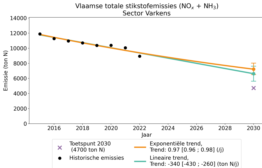
Figuur 21: Verloop van de jaarlijkse totale stikstofemissies ( \text{NO}_x + \text{NH}_3 ) voor de sector Varkens in Vlaanderen (in ton N). Zwarte punten: gerapporteerde jaarlijkse emissies voor de historische jaren. Groene en oranje lijn: lineaire respectievelijk exponentiële regressie door de punten voor de periode 2015-2022. Groene en oranje punt in 2030: projectie van de emissies volgens een lineaire respectievelijke exponentiële trend, met betrouwbaarheidsinterval (2-sigma onzekerheid). Paarse kruis: toetspunt voor 2030.
