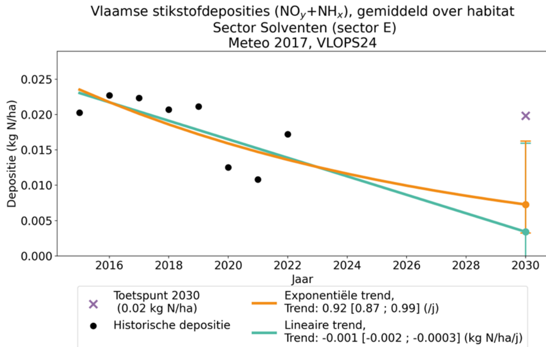
Figuur 37: Verloop van de jaarlijkse Vlaamse stikstofdeposities ( \text{NO}_y + \text{NH}_x ) gemiddeld over habitats in Vlaanderen voor de sector Solventen (sector E) (in kg N/ha/j). Zwarte punten: gemodelleerde jaarlijkse deposities voor de historische jaren. Groene en oranje lijn: lineaire respectievelijk exponentiële regressie door de punten. Groene en oranje punt in 2030: projectie van de depositie volgens een lineaire respectievelijke exponentiële trend, met betrouwbaarheidsinterval (2-sigma onzekerheid). Paarse kruis: toetspunt voor 2030.
