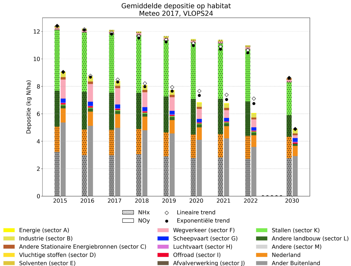
Figuur 27: Opbouw van de jaarlijkse deposities op stikstofgevoelige habitats binnen SBZ-H (in kg N/ha/j) voor zowel NH x - (links, gestippelde balken) als NO y -depositie (rechtse niet-gestippelde balken). De plot toont zowel de resultaten voor historische jaren als voor het toetspunt voor 2030. Deposities zijn berekend op basis van VLOPS24 en meteo 2017. De open ruitjes tonen per jaar wat de depositie zou zijn bij een lineaire evolutie tussen 2015 en het toetspunt, de gevulde bolletjes tonen per jaar wat de depositie zou zijn bij een exponentiële evolutie tussen 2015 en het toetspunt. Voor meer detail verwijzen we naar de tekst.
