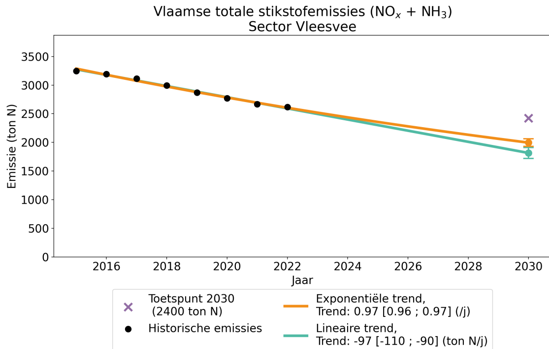
Figuur 19: Verloop van de jaarlijkse totale stikstofemissies ( \text{NO}_x + \text{NH}_3 ) voor de sector Vleesvee in Vlaanderen (in ton N). Zwarte punten: gerapporteerde jaarlijkse emissies voor de historische jaren. Groene en oranje lijn: lineaire respectievelijk exponentiële regressie door de punten voor de periode 2015-2022. Groene en oranje punt in 2030: projectie van de emissies volgens een lineaire respectievelijke exponentiële trend, met betrouwbaarheidsinterval (2-sigma onzekerheid). Paarse kruis: toetspunt voor 2030.
