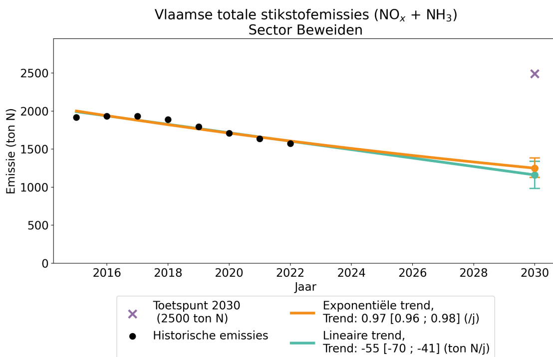
Figuur 23: Verloop van de jaarlijkse totale stikstofemissies ( \text{NO}_x + \text{NH}_3 ) voor de sector Beweiden in Vlaanderen (in ton N). Zwarte punten: gerapporteerde jaarlijkse emissies voor de historische jaren. Groene en oranje lijn: lineaire respectievelijk exponentiële regressie door de punten voor de periode 2015-2022. Groene en oranje punt in 2030: projectie van de emissies volgens een lineaire respectievelijke exponentiële trend, met betrouwbaarheidsinterval (2-sigma onzekerheid). Paarse kruis: toetspunt voor 2030.
