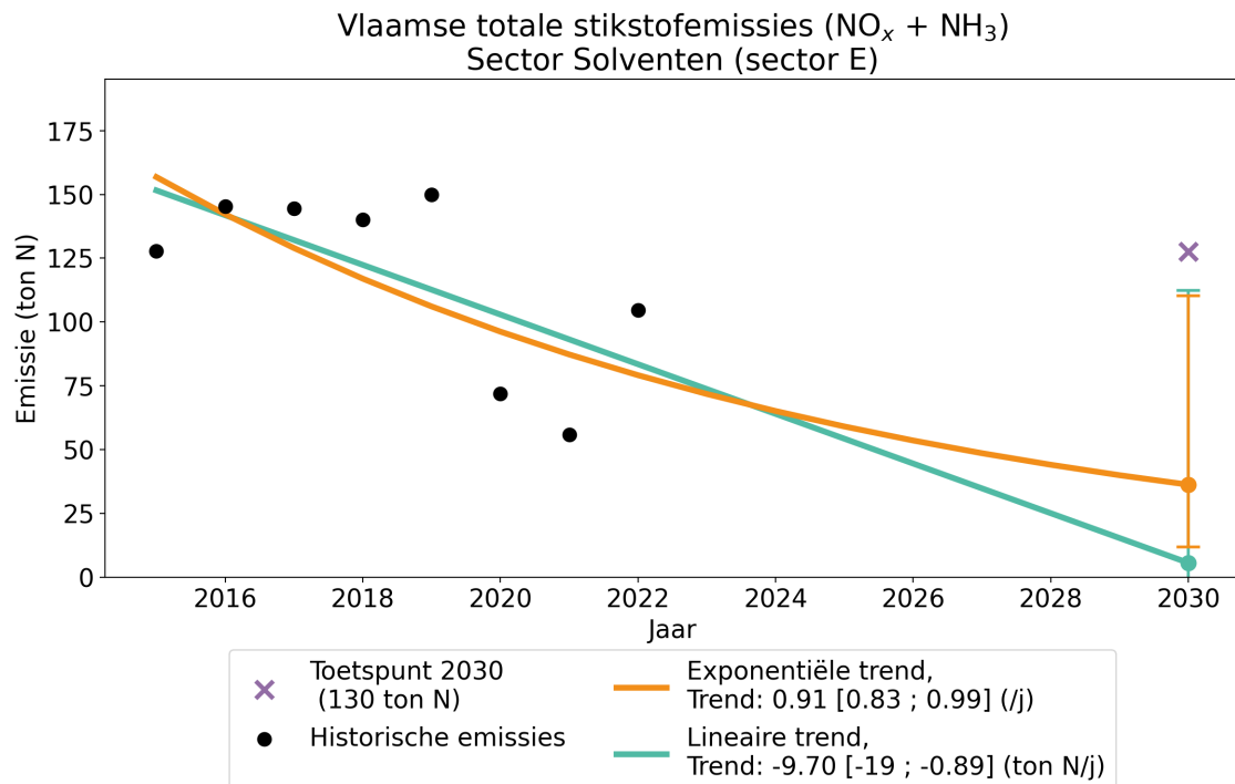
Figuur 7: Verloop van de jaarlijkse totale stikstofemissies ( \text{NO}_x + \text{NH}_3 ) voor de sector Solventen (sector E) in Vlaanderen (in ton N). Zwarte punten: gerapporteerde jaarlijkse emissies voor de historische jaren. Groene en oranje lijn: lineaire respectievelijk exponentiële regressie door de punten voor de periode 2015-2022. Groene en oranje punt in 2030: projectie van de emissies volgens een lineaire respectievelijk exponentiële trend, met betrouwbaarheidsinterval (2-sigma onzekerheid). Paarse kruis: toetspunt voor 2030.
