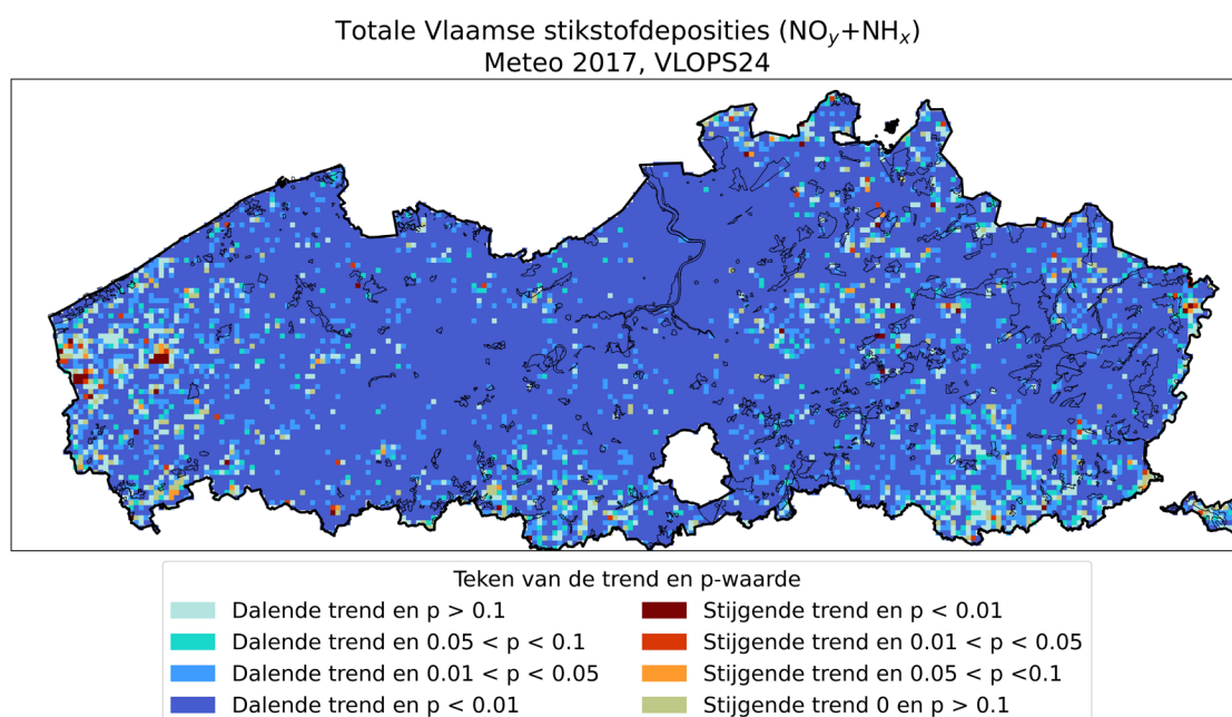
Figuur 48: Lineaire trend van de Vlaamse jaarlijkse stikstofdeposities ( \text{NO}_y + \text{NH}_x ) op 1 km bij 1 km resolutie in de periode 2015 – 2022, zoals gemodelleerd door het VLOPS model. De bovenste figuur geeft de jaarlijkse trend (in kg N/ha/jaar), de onderste figuur visualiseert het teken van de trend en de p-waarde in één figuur. De dikke zwarte lijn geeft de buitengrenzen van Vlaanderen weer, de dunne lijnen de locaties van de Habitatrichtlijngebieden (SBZ-H).
