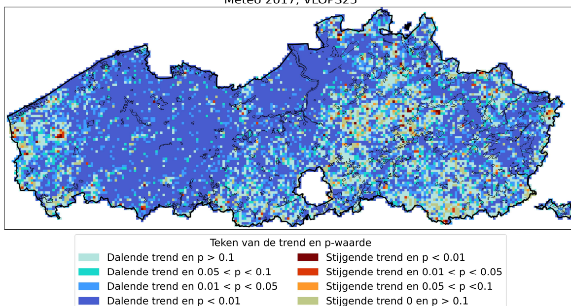
Figuur 51: Lineaire trend van de Vlaamse NH x -deposities op 1 km bij 1 km resolutie in de periode 2015 – 2023, zoals gemodelleerd door het VLOPS model. De bovenste figuur geeft de jaarlijkse trend (in kg/ha/jaar), de onderste figuur visualiseert het teken van de trend en de p-waarde in één figuur. De dikke zwarte lijn geeft de buitengrenzen van Vlaanderen weer, de dunne lijnen de locaties van de Natura 2000 gebieden.
