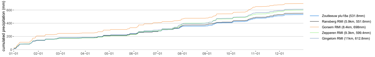
Zoutleeuw plu18a cumulative precipitation in 2025
