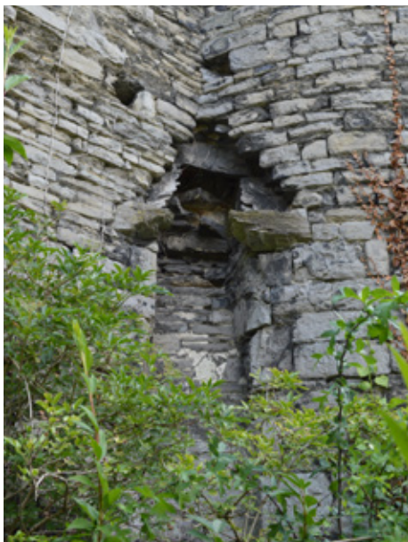
Latrine met schuine afloop in de keel van de ronde hoektoren, waarvan de schacht is opgevuld met steenpuin.
