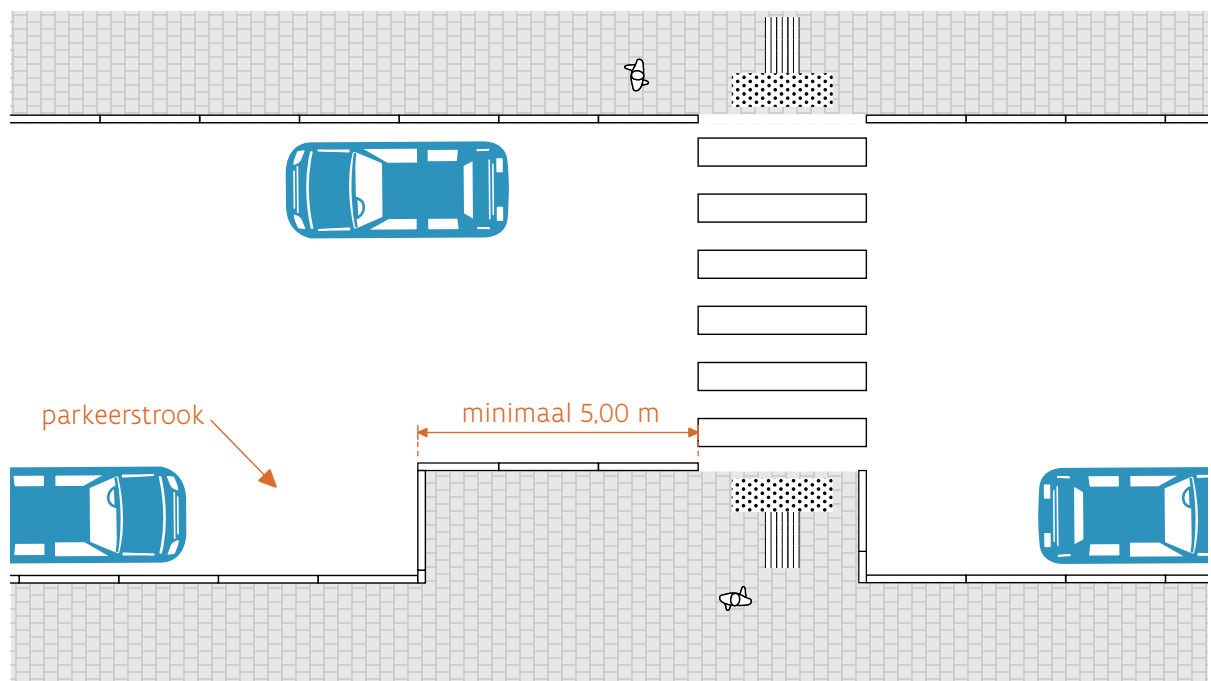
Figuur 5: Voetpaduitstulping
