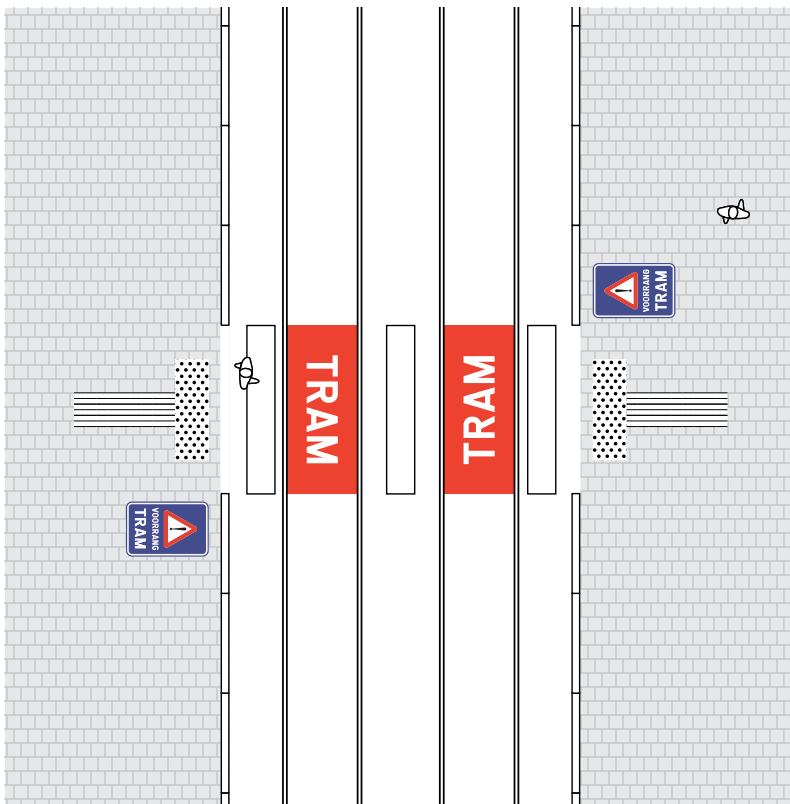
Figuur 14: Tramspoor met zebrapad
