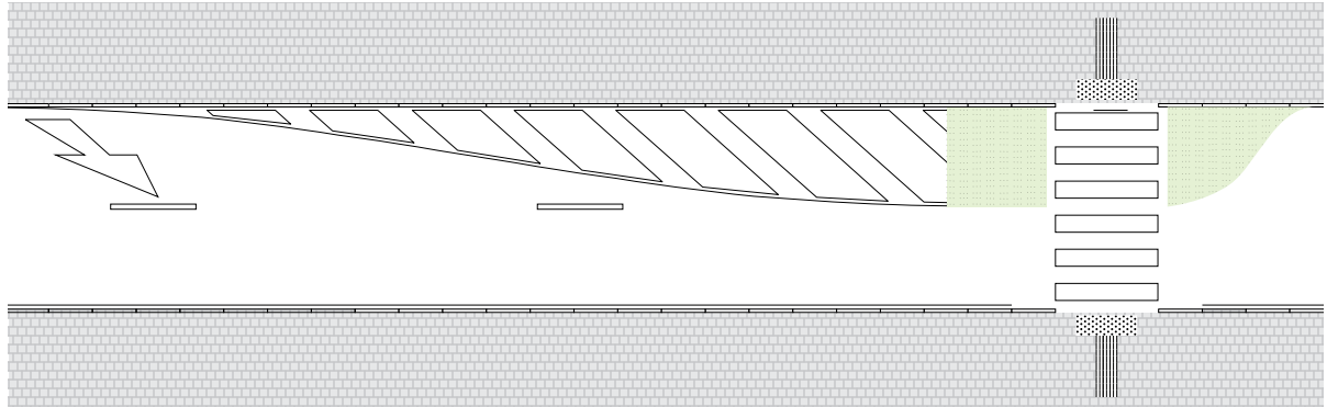
Figuur 4: Rijbaanversmalling
