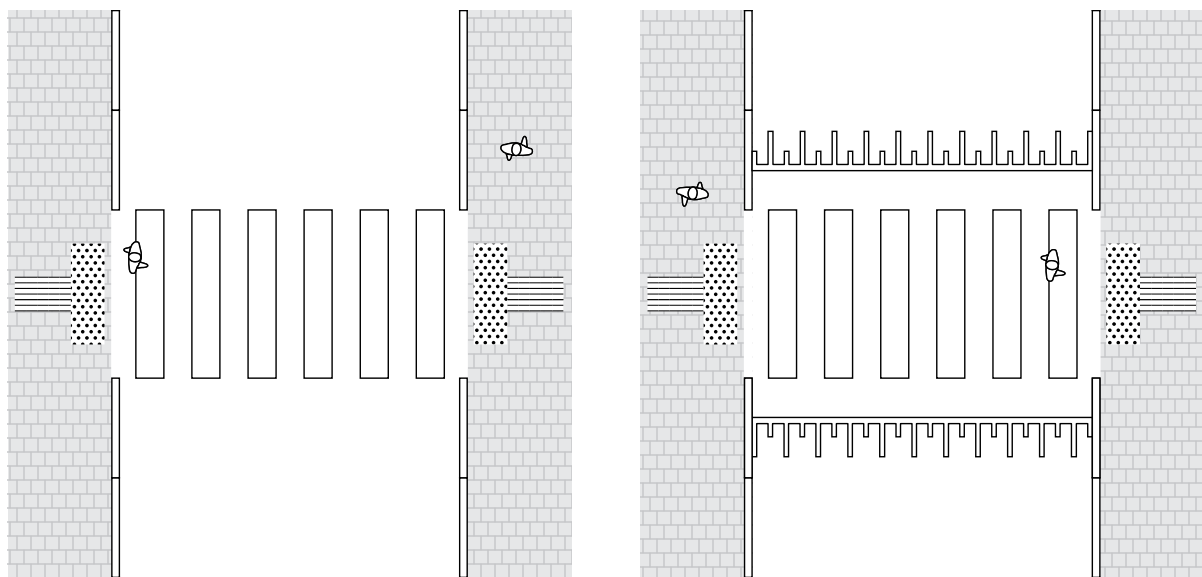
Figuur 8: Zebrapad en zebrapad op verkeersplateau
