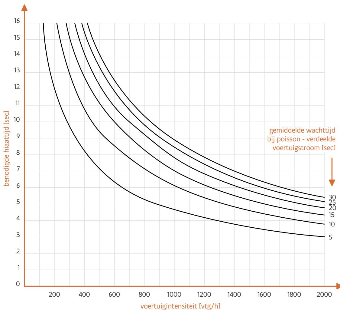
Figuur 2: Benodigde hiaattijd in functie van de voertuigintensiteit die in één oversteekbeweging moet worden gekruist. 5
