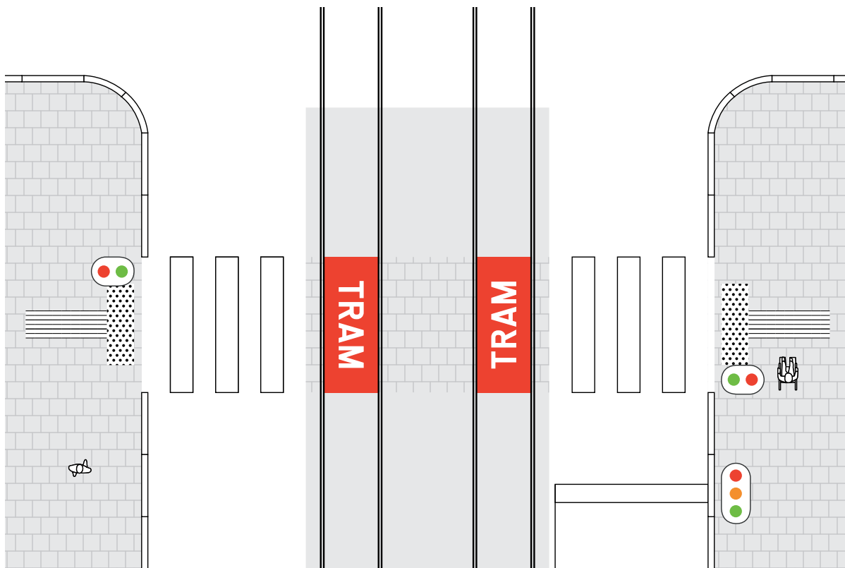
Figuur 13: Tramspoor met lichtengeregelde oversteekplaats
