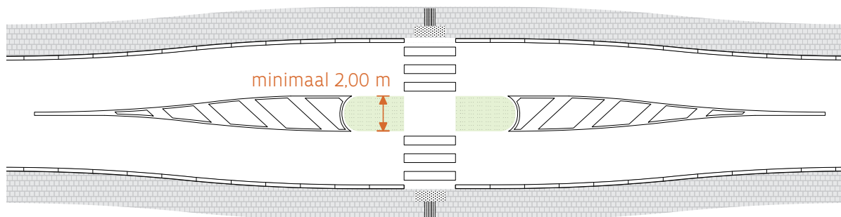
Figuur 3: Middeneiland
