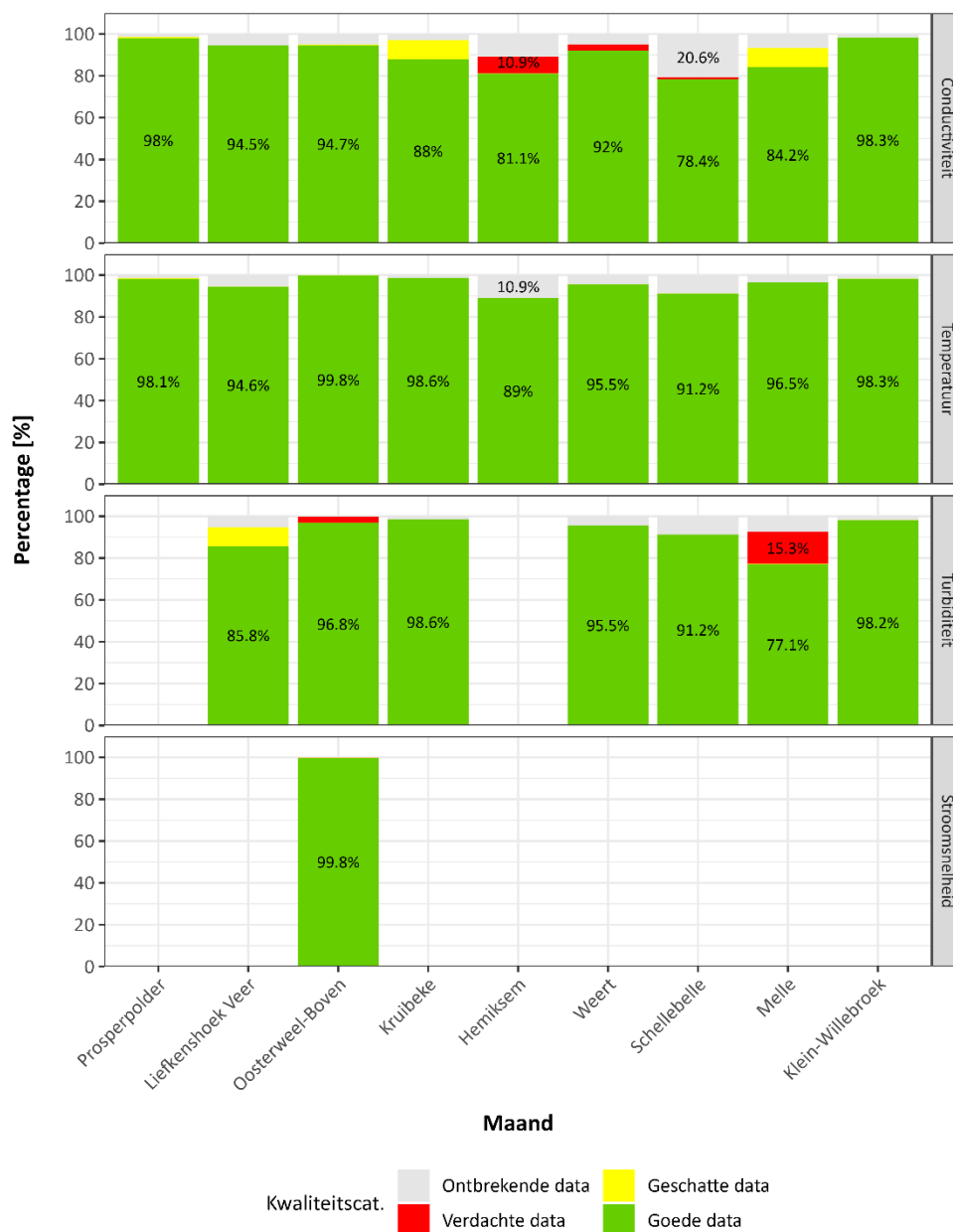
Figuur 120 – Percentage van de datakwaliteitscategorieën per parameter en per station voor de continue metingen fysische parameters in 2025, voorgesteld in Figuur 119. Percentages worden getoond wanneer groter dan 10%. In Prosperpolder en Hemiksem wordt er geen turbiditeit gemeten. Stroomsnelheid wordt enkel in Oosterweel-Boven gemeten
