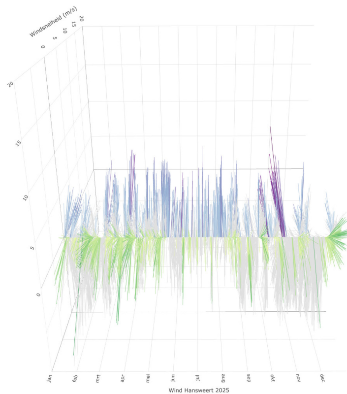
Figuur 13 – Windrichting en -snelheid in Hansweert doorheen 2025 met aanduiding van de noordwestenwinden (opwaaiing, blauw → paars) en oostenwinden (afwaaiing, geel → groen) (Bron: Rijkswaterstaat).
