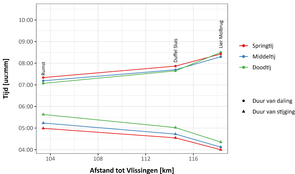
Figuur 7 – Duur van stijging en daling bij middeltij, springtij en doodtij in 2025 voor de Beneden-Nete.
