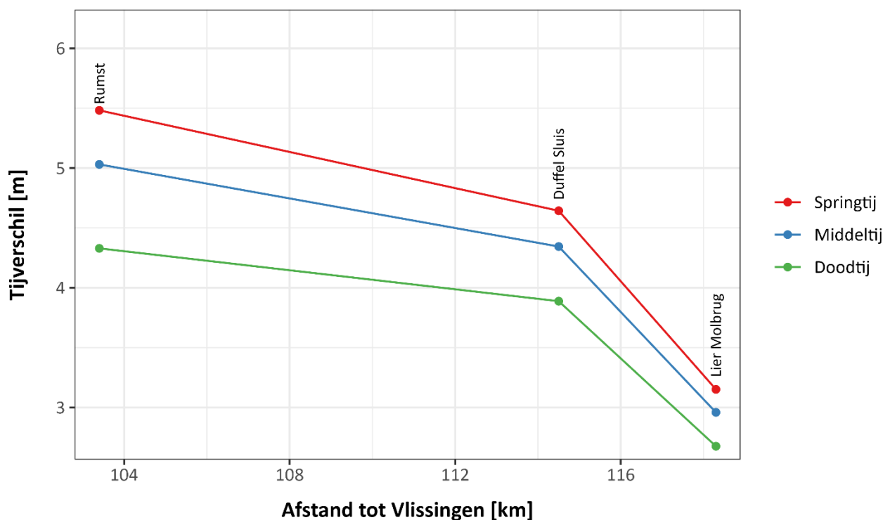
Figuur 6 – Gemiddeld tijvershil (GTV) bij middeltij, springtij en doodtij in 2025 voor de Beneden-Nete.
