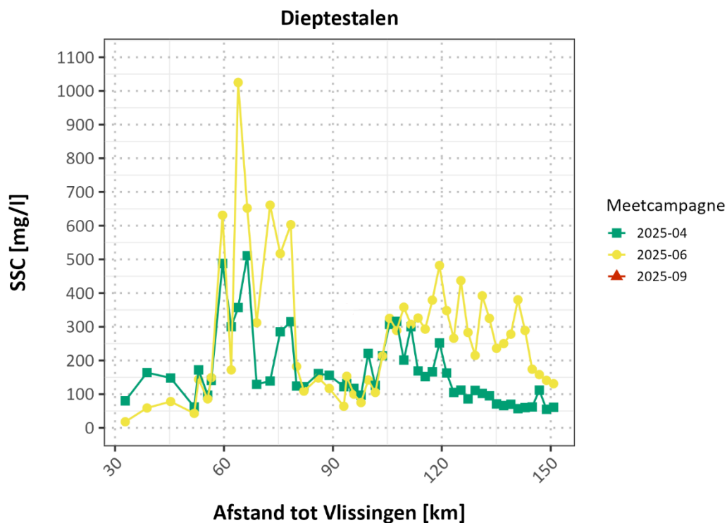
Figuur 67 – Sedimentconcentratie aan de bodem bij half-tij-eb langs de volledige Zeeschelde
