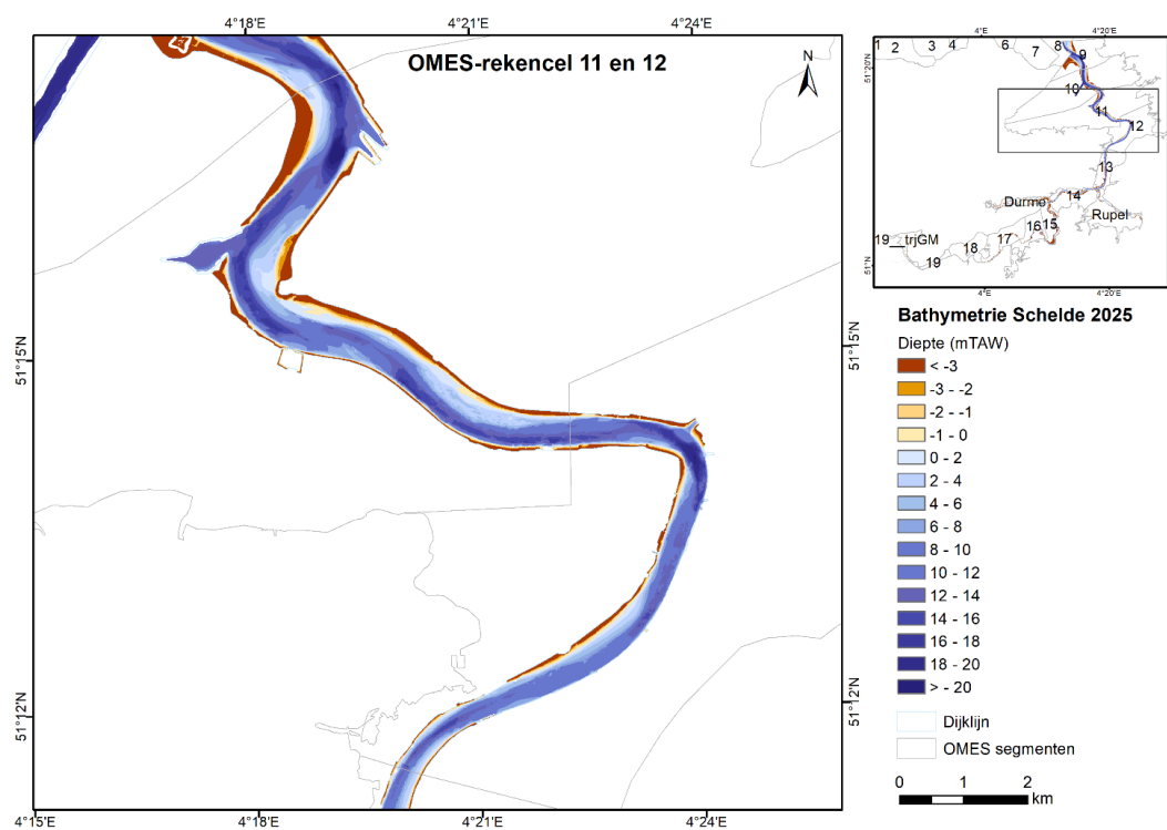
Figuur 124 – Topo-bathymetrie 2025 Zeeschelde: OMES-segmenten 11 en 12.
