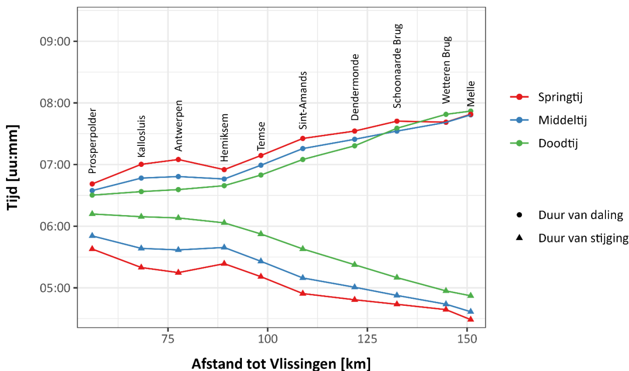
Figuur 4 – Zeeschelde: gemiddelde duur van stijging en daling bij middeltij, springtij en doottij in 2025 t.o.v. de afstand in km tot de monding te Vlissingen.
