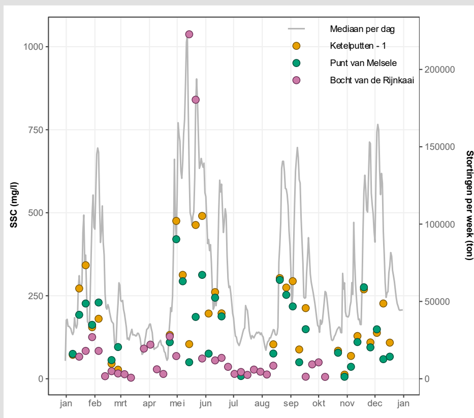
Figuur 52 – Variatie van SSC te Oosterweel en wekelijkse storthoeveelheid slib per stortlocatie
