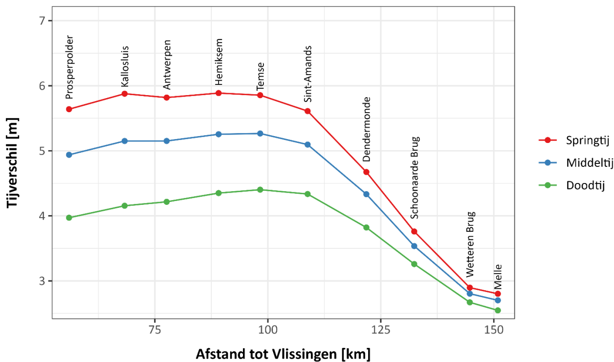
Figuur 3 – Zeeschelde: gemiddeld tijverschil (GTV) bij middeltij, springtij en doodtij in 2025 t.o.v. de afstand in km tot de monding te Vlissingen.
