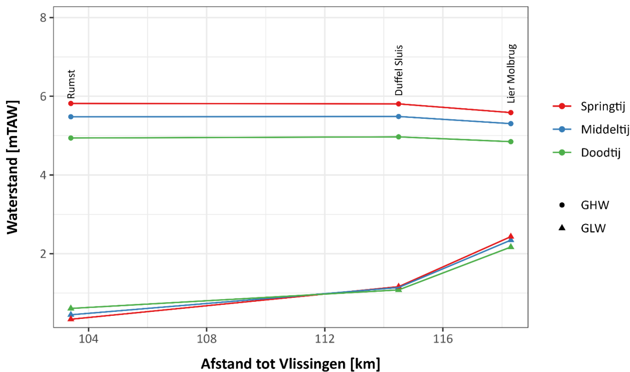
Figuur 5 – Gemiddeld hoogwater (GHW) en gemiddeld laagwater (GLW) bij middeltij, springtij en doottij in 2025 voor de Beneden-Nete.
