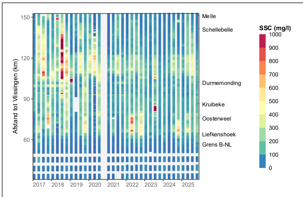
Figuur 68 – Sedimentconcentratie nabij het oppervlak (mg/l) bij half-tij-eb langs de Zeeschelde (interpolatietechniek: inverse distance weight, zoekradius Y-as: 2 km)
