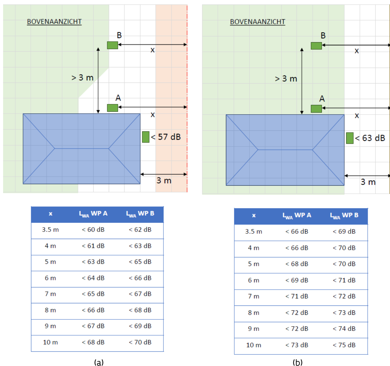
Figuur 10: Maximale geluidsvermogenenniveaus van de buitenunit voor diverse posities in de tuin (positie A en B) om te voldoen aan de vooropgestelde geluidsvoorwaarde van 45 dB(A) L_{Aeq,1min} overdag ter hoogte van de perceelsgrens. x is de kleinste afstand tot de dichtstbijzijnde perceelsgrens, in dit voorbeeld is hiervoor de perceelsgrens rechts gekozen. De geluidsbron wordt verondersteld op 0,75 m (2/3 van de hoogte van de unit) en de geluidsdruk werd geëvalueerd op de perceelsgrens op 1,5 m hoogte. In situatie (a) zijn geen afsluitingen tussen de tuinen die een voldoende massa hebben om te zorgen voor afscherming. In situatie (b) is er een volledig gesloten afsluiting met hoogte 1,8 m en oppervlaktemassa \geq 10 \text{ kg/m}^2 aanwezig over de volledige lengte van de perceelsgrens. Daarnaast wordt voor de 2 situaties ook het maximale geluidsvermogen weergegeven voor een buitenunit geplaatst bij de zijgevel op 3 m van de perceelsgrens. Merk op dat in bovenstaande figuur links geen perceelsgrens ingetekend is. Men moet de afstanden in bovenstaande figuur dus ook steeds nagaan voor de linkerzijde (gespiegeld). De groene arcering loopt in werkelijkheid niet door tot aan de linkerperceelsgrens! Ook daar zal een rode en witte zone aanwezig zijn.
