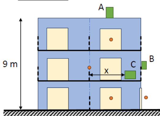
Figuur 19: Maximale geluidsvermogeniveaus van de buitenunit van het appartement op de eerste verdieping voor een plaatsing op het dak (A), aan de gevel (B) of op het balkon (uit beton of massief hout) van het appartement (C) om te voldoen aan de vooropgestelde geluidsvoorwaarde 45 dB(A) L_{Aeq,1min} overdag. De geluidsdruk werd geëvalueerd voor de opengaande ramen en terrassen van de naburige appartementen. x is de afstand van de buitenunit tot het dichtstbijzijnde opengaande raam of een terras waar je kan verblijven.
