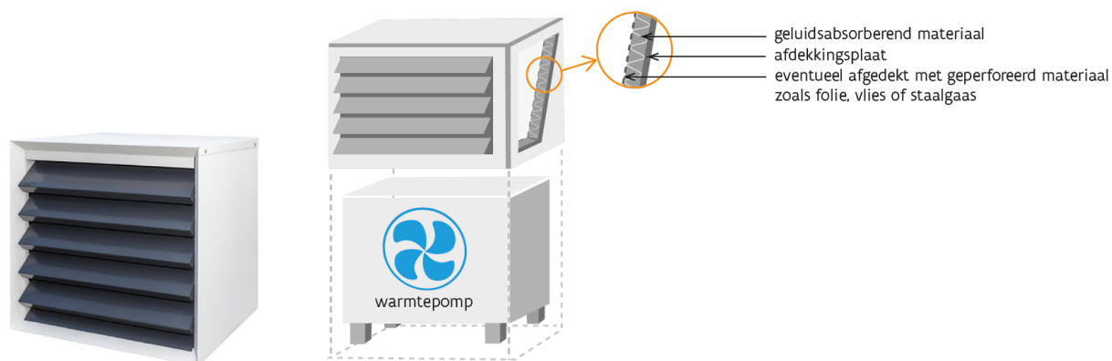
Figuur 9: Voorbeeld van een akoestische omkasting met doorsnede.
