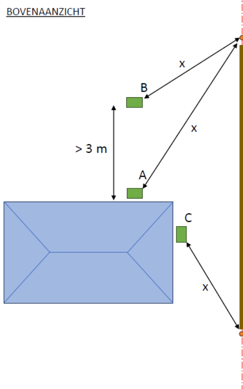
Figuur 12: Maximale geluidsvermogen-niveaus van de buitenunit voor diverse posities in de tuin (positie A, B en C) om te voldoen aan de vooropgestelde geluidsvoorwaarde van 45 dB(A) L_{Aeq,1min} overdag op de perceelsgrens. x is de afstand van de buitenunit tot het dichtstbijzijnde punt op de perceelsgrens zonder afsluiting.
