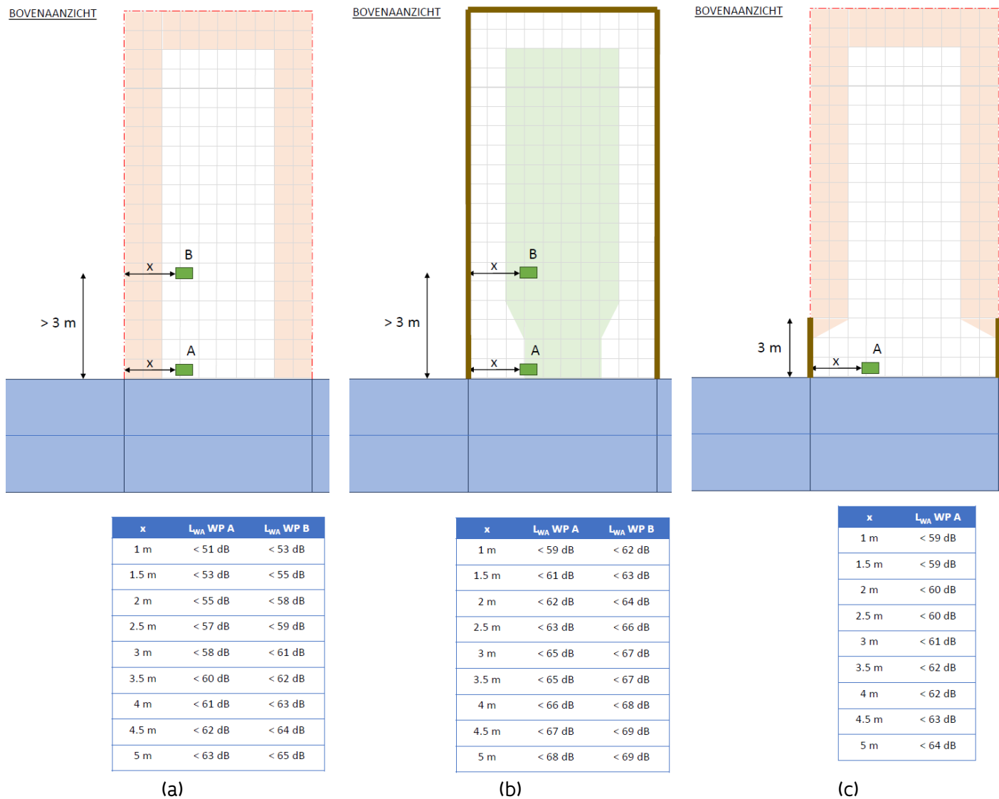
Figuur 15: Maximale geluidsvermogenenniveaus van de buitenunit voor diverse posities in de achtertuin (positie A en B 35 ) om te voldoen aan de vooropgestelde geluidsvoorwaarde 45 dB(A) L_{Aeq,1min} overdag. x is de kleinste afstand tot de dichtstbijzijnde perceelsgrens. De geluidsbron wordt verondersteld op 0,75 m (2/3 van de hoogte van de unit) en de geluidsdruk werd geëvalueerd op de perceelsgrens op 1,5 m hoogte. In situatie (a) zijn geen afsluitingen tussen de tuinen die een voldoende massa hebben om te zorgen voor afscherming. In situatie (b) is een volledig gesloten afsluiting met hoogte 1,8 m en oppervlaktemassa \geq 10 \text{ kg/m}^2 rondom de volledige tuin 36 en in situatie (c) zijn volledig gesloten afsluitingen met lengte 3 m, hoogte 1,8 m en oppervlaktemassa \geq 10 \text{ kg/m}^2
