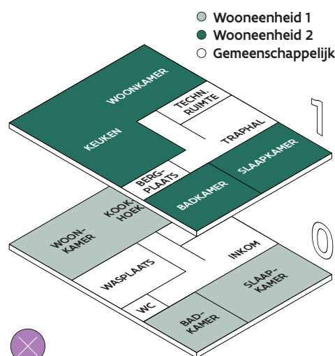
FIGUUR 2 Twee wooneenheden met enkel de circulatieluimte en technische ruimte gemeenschappelijk, voldoen strikt genomen niet aan de voorwaarde 'ondergeschikte wooneenheid'.
